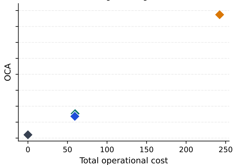
Noisy external
