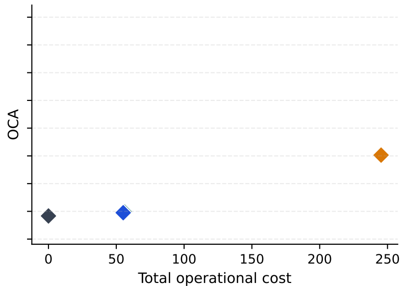
Noisy external
