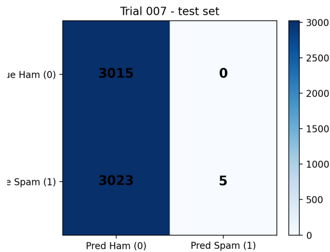
5.1. ábra: A 7. kísérlet konfúziós mátrixa. A modell egyoldalú döntése alapján a teszthalmazon öt darab kivétellel az összes üzenet helytelenül valódi üzenetként került felcímkézésre.
