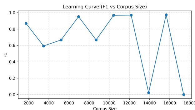
5.4. ábra: Instabil modell növekményes tanulási görbéje az F1-érték szerint, a második fázisban.
