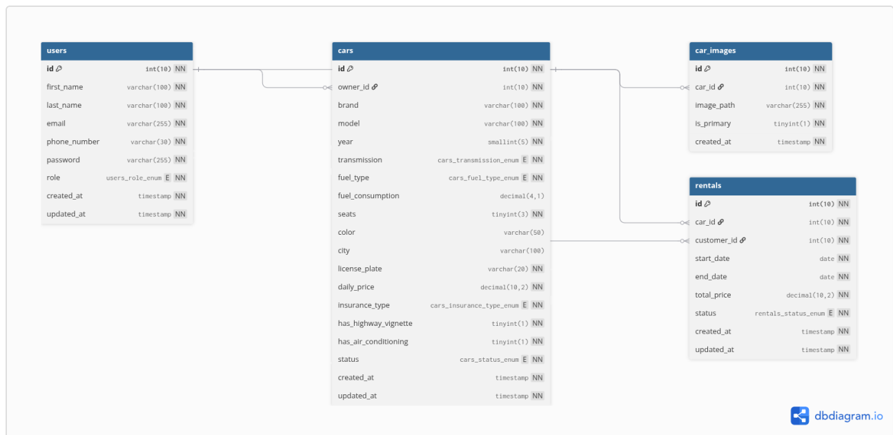
1. ábra — Az adatbázis struktúrája (dbdiagram.io).
