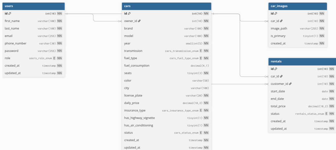
1. ábra — Az adatbázis struktúrája (dbdiagram.io).
