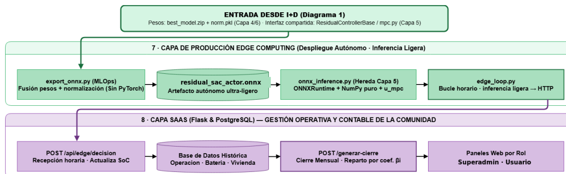
Figura 5.5: Arquitectura de la plataforma, parte 2: producción edge (exportación ONNX, inferencia ligera y bucle horario) y capa SaaS (recepción de decisiones, histórico y cierres mensuales).
