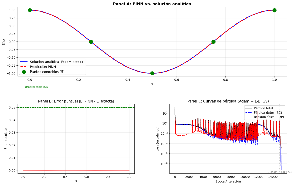
Figura 4.1. Validación PINN-SIREN para Helmholtz 1D. Panel A: comparación entre la predicción de la red y la solución analítica E_{\text{exacta}}(x) = \cos(kx) en 1,000 puntos uniformes en [0, 1] . Panel B: error puntual |\hat{E}(x) - E_{\text{exacta}}(x)| . Panel C: curva de pérdida total durante las fases Adam y L-BFGS; la transición a la época 15,000 es visible como una caída abrupta. Error L^2 = 0.006\% , R^2 = 1.000000 . GPU: NVIDIA RTX 5050, SEED = 42.
