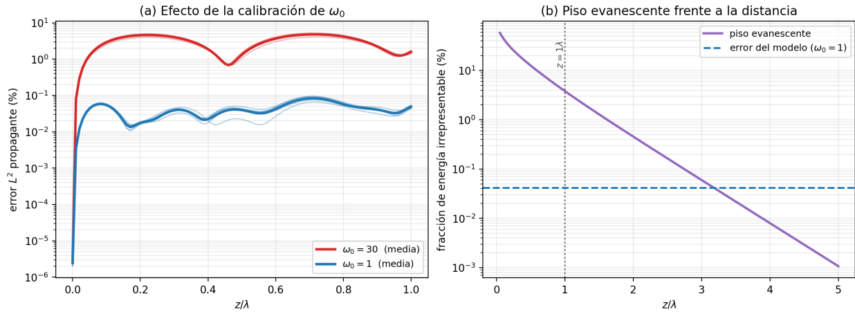
Figura 4.6. Resultados de NB03 modal. (a) Error L^2 propagante a lo largo de la propagación para las cinco pantallas, con \omega_0 = 30 (rojo) y \omega_0 = 1 (azul); las curvas tenues son las pantallas individuales y las gruesas su promedio. La separación es de aproximadamente dos órdenes de magnitud en todo el intervalo. (b) Fracción de energía irrepresentable por la base modal —el piso evanescente— frente a la distancia de propagación, en escala logarítmica, junto al error medio del modelo calibrado. Cómo leerla: en \tilde{z} = 1\lambda el piso es 92 veces mayor que el error del modelo, de modo que la métrica de campo completo mide la física irrepresentable y no el ajuste de la red. El piso decae con la distancia y cruzaría el nivel de error aquí medido alrededor de \tilde{z} \approx 3.2\lambda si ese error se mantuviera constante, extrapolación que este trabajo no verifica: el modelo sólo se validó en \tilde{z} = 1\lambda , y el ensayo de extensión a 2\lambda (§4.4.11) muestra que el error crece con la distancia. Fuentes: results/nb03_modal_multiseed_z1_omega1_12_curves.npz y results/nb03_angular_spectrum_reference_z1_corr0.10.npz.
