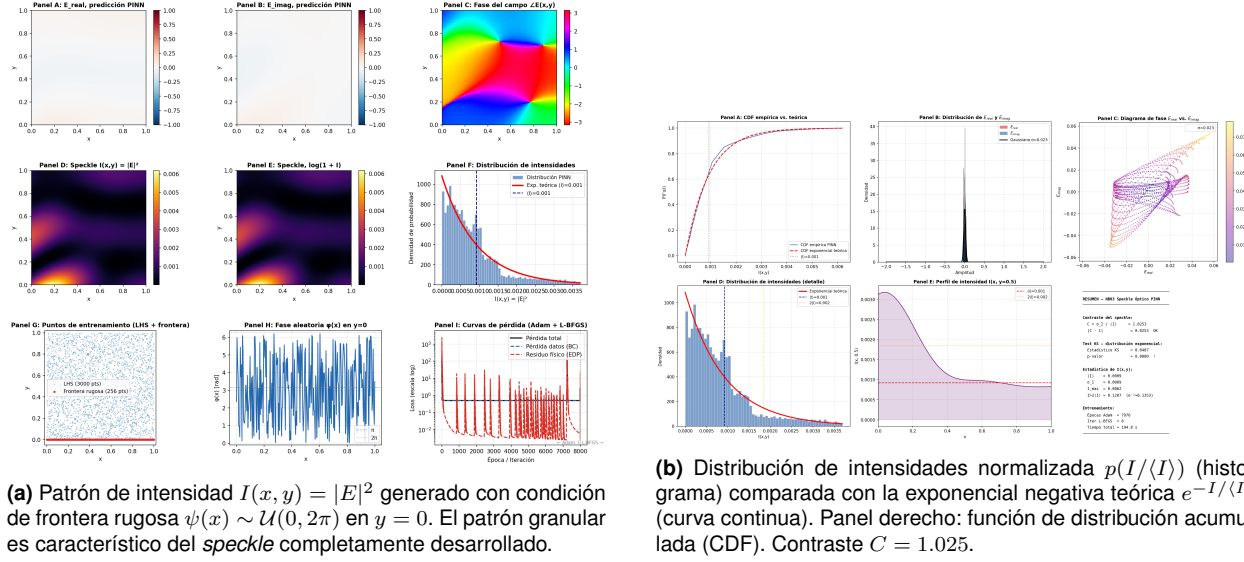
Figura 4.5. Simulación de speckle óptico con PINN-SIREN (NB03).
