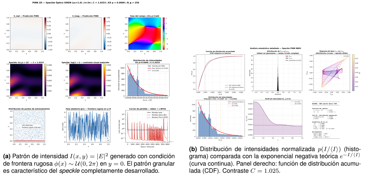
Figura 4.5. Simulación de speckle óptico con PINN-SIREN (NB03).
