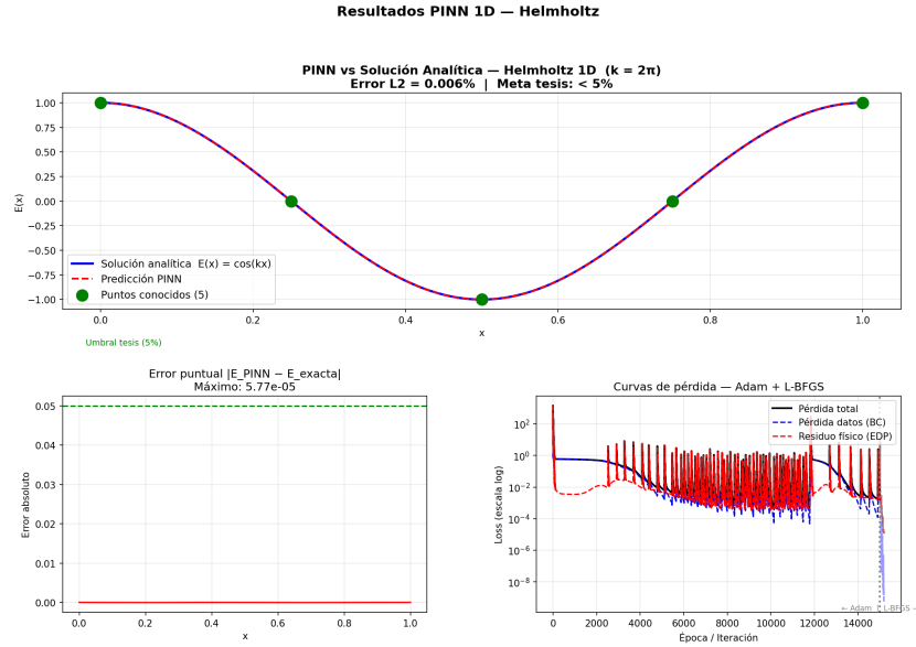
Figura 1. Validación PINN-SIREN para Helmholtz 1D. (a) Comparación entre la predicción de la red y la solución analítica E_{\text{exacta}}(x) = \cos(kx) en 1,000 puntos uniformes en [0, 1] . (b) Error puntual |\hat{E}(x) - E_{\text{exacta}}(x)| . Error L^2 = 0,006\% , R^2 = 1,000000 . GPU: NVIDIA RTX 5050, SEED = 42.
