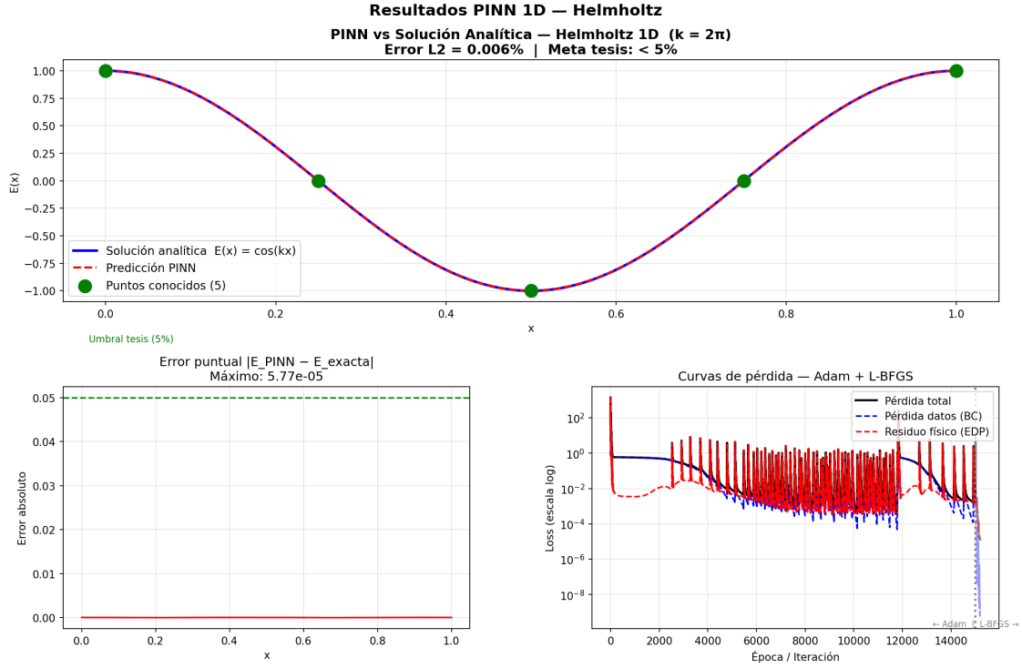
Figura 1: Validación PINN-SIREN para Helmholtz 1D. (a) Comparación entre la predicción de la red y la solución analítica E_{exacta}(x) = \cos(kx) en 1,000 puntos uniformes en [0, 1] . (b) Error puntual |\hat{E}(x) - E_{exacta}(x)| . Error L^2 = 0,006\% , R^2 = 1,000000 . GPU: NVIDIA RTX 5050, SEED = 42.
