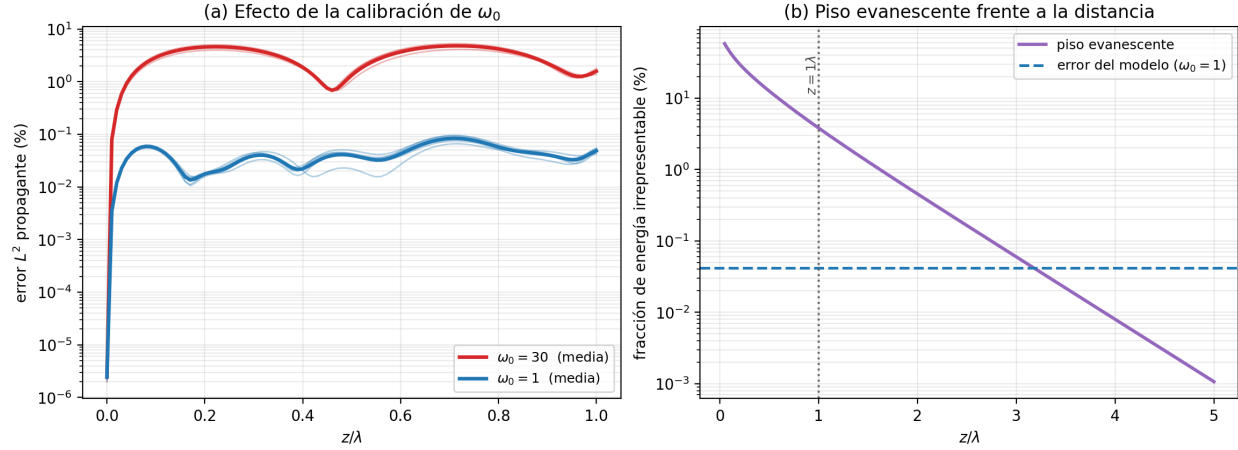
Figura 4.5. Resultados de NB03 modal. (a) Error L^2 propagante a lo largo de la propagación para las cinco pantallas, con \omega_0 = 30 (rojo) y \omega_0 = 1 (azul); las curvas tenues son las pantallas individuales y las gruesas su promedio. La separación es de aproximadamente dos órdenes de magnitud en todo el intervalo. (b) Fracción de energía irrepresentable por la base modal —el piso evanescente— frente a la distancia de propagación, en escala logarítmica, junto al error medio del modelo calibrado. Cómo leerla: en \tilde{z} = 1\lambda el piso es 92 veces mayor que el error del modelo, de modo que la métrica de campo completo mide la física irrepresentable y no el ajuste de la red. El piso decae con la distancia y cruzaría el nivel de error aquí medido alrededor de \tilde{z} \approx 3.2\lambda si ese error se mantuviera constante, extrapolación que este trabajo no verifica: el modelo sólo se validó en \tilde{z} = 1\lambda , y el ensayo de extensión a 2\lambda (§4.4.9) muestra que el error crece con la distancia. Fuentes: results/nb03_modal_multiseed_z1_omega1_12_curves.npz y results/nb03_angular_spectrum_reference_z1_corr0.10.npz .
