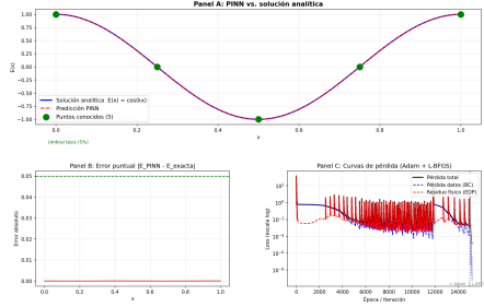
Fig. 1. Validación PINN-SIREN para Helmholtz 1D. (a) Comparación entre la predicción de la red y la solución analítica E_{\text{exacta}}(x) = \cos(kx) en 1,000 puntos uniformes en [0, 1] . (b) Error puntual |E(x) - E_{\text{exacta}}(x)| . Error L^2 = 0,006\% , R^2 = 1,000000 . GPU: NVIDIA RTX 5050, SEED = 42.
