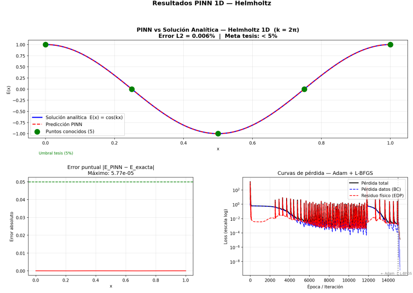
Figura 1. Validación PINN-SIREN para Helmholtz 1D. (a) Comparación entre la predicción de la red y la solución analítica E_{exacta}(x) = \cos(kx) en 1,000 puntos uniformes en [0, 1] . (b) Error puntual |\hat{E}(x) - E_{exacta}(x)| . Error L^2 = 0,006\% , R^2 = 1,000000 . GPU: NVIDIA RTX 5050, SEED = 42.
