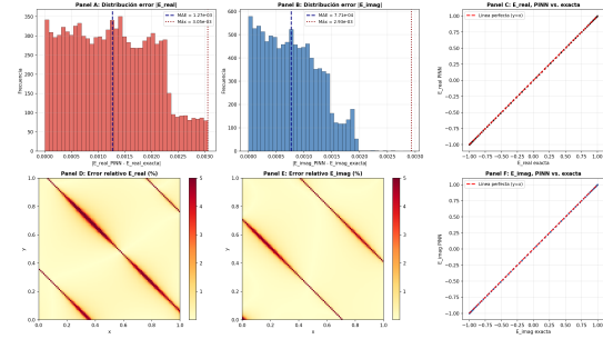
Fig. 4. Métricas adicionales de entrenamiento NB02. Paneles A-B: distribución del error absoluto |E_{\text{real}} - \hat{E}_{\text{real}}| y |E_{\text{imag}} - \hat{E}_{\text{imag}}| . Paneles C, F: dispersión de la predicción PINN contra la solución exacta para cada componente. Paneles D-E: error relativo puntual (%) en la malla 100 \times 100 ; los valores más altos se concentran en bandas anti diagonales ( x + y \approx \text{const.} ) donde la solución exacta cruza por cero, no en las esquinas del dominio. La curva de pérdida de entrenamiento se muestra en el Panel C3 de la Figura 3.
