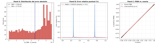
Fig. 2. Métricas adicionales de entrenamiento NB01. Panel A: distribución del error absoluto |E(x) - E_{\text{exact}}(x)| . Panel B: error relativo puntual (%). Panel C: dispersión de la predicción PINN contra la solución exacta, con la línea y = x como referencia de ajuste perfecto.
