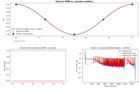
Fig. 1. Validación PINN-SIREN para Helmholtz 1D. Panel A: comparación entre la predicción de la red y la solución analítica E_{\text{exact}}(x) = \cos(kx) en 1,000 puntos uniformes en [0, 1] . Panel B: error puntual |E(x) - E_{\text{exact}}(x)| . Panel C: curva de pérdida total durante las fases Adam y L-BFGS. Error L^2 = 0,006\% , R^2 = 1,000000 . GPU: NVIDIA RTX 5050, SEED = 42.
