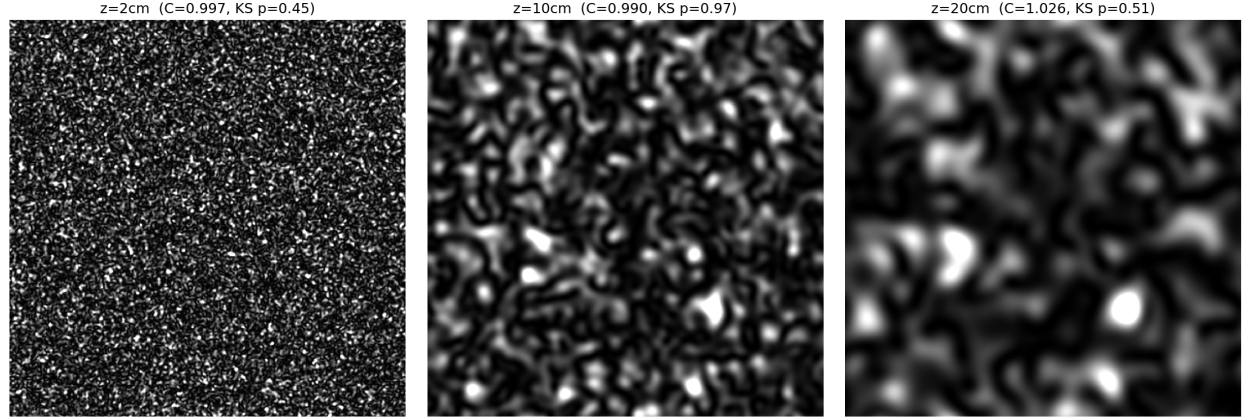
Figura 4.5. Patrones de speckle generados estadísticamente (NB03) a z = 2, 10 y 20 cm. El tamaño de grano crece con la distancia, consistente con \text{grano} \approx \lambda z/D . Contraste C y p -valor KS (muestra decorrelacionada) indicados por panel; ver Tabla 4.5 para las 10 distancias completas.
