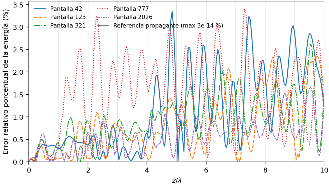
Figura 4.10. Error relativo porcentual de la energía, ecuación (4.5), evaluado sobre la predicción de la PINN en las cinco pantallas a lo largo de los 201 planos. La línea gris es la referencia restringida al subespacio propagante, que conserva la energía a precisión de máquina y sirve de línea base. Las líneas verticales tenues marcan las nueve interfaces. Generada por scripts/build/figuras_nb03d_z10.py .
