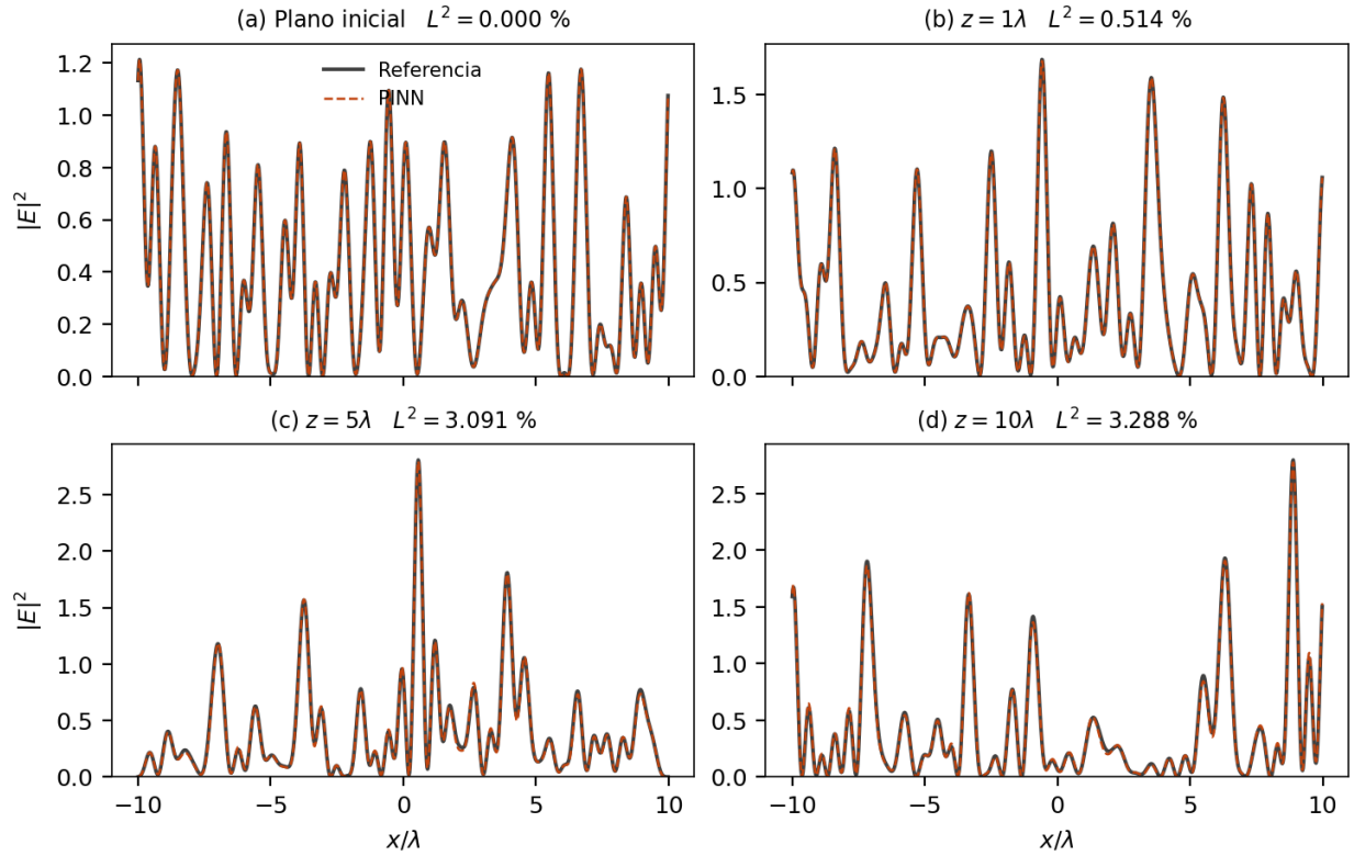
Figura 4.8. Perfiles transversales de intensidad |E|^2 de la pantalla 42 en cuatro planos del recorrido, con la referencia restringida al subespacio propagante en trazo continuo y la PINN-SIREN modal en trazo discontinuo. La disposición reproduce la de la figura 5.2 de Hernández Nolasco (2003), con una diferencia obligada: aquel trabajo simula en tres dimensiones y puede representar cada plano como una superficie sobre (x, y) , mientras que el dominio de esta formulación tiene una única dimensión transversal, de modo que cada plano es un perfil. Los dos campos se superponen en el mismo eje, al modo de las figuras 3 y 4 de Andrés-Zárate et al. (2019), para que la comparación sea directa. El panel (a) exhibe la condición de Cauchy dura: el error es idénticamente nulo en z = 0 porque el plano inicial no se aprende sino que se impone por construcción. Los tres restantes muestran la maduración del speckle , con una estructura transversal fina que evoluciona hacia granos más escasos y de mayor amplitud. El valor de 3.288 % del panel (d) coincide con el de la pantalla 42 en la Tabla 4.17, como debe. Generada por scripts/build/figuras_nb03d_z10.py .
