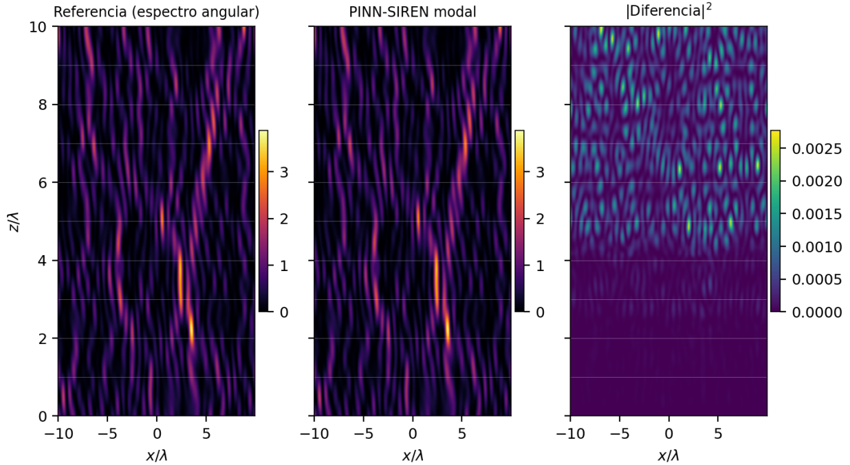
Figura 4.9. Mapas de intensidad |E|^2 sobre el plano de propagación completo (\tilde{x}, \tilde{z}) para la pantalla 42, con 0 \leq z \leq 10\lambda y -10 \leq \tilde{x} \leq 10 . Izquierda, la referencia por espectro angular restringida al subespacio propagante; centro, la PINN-SIREN modal, en la misma escala de color; derecha, el módulo al cuadrado de su diferencia, en escala propia. Las líneas horizontales tenues marcan las nueve interfaces entre los diez bloques de 1\lambda . Los dos primeros paneles son indistinguibles a simple vista: el pico de la diferencia vale 2.77 \times 10^{-3} frente a una intensidad máxima de 3.88, esto es, el 0.07% del pico. El tercer panel muestra dónde reside ese error, y es su información propia: la discrepancia es despreciable por debajo de z \approx 3\lambda y crece de forma visible a partir del quinto bloque, que es justamente donde empiezan las redes entrenadas en esta extensión y donde se acumula lo transferido por las anteriores. La presentación sigue el formato de sección transversal a lo largo de la propagación empleado por Hernández Nolasco (2003). Generada por scripts/build/figuras_nb03d_z10.py a partir de results/nb03_distance_pilot/z10_screen42_net42_adaptive_slabs_v1/adaptive_slabs_z10.npz .
