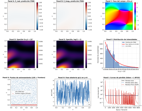
(a) Patrón de intensidad I(x, y) = |E|^2 generado con condición de frontera rugosa \psi(x) \sim \mathcal{U}(0, 2\pi) en y = 0 . El patrón granular es característico del speckle completamente desarrollado.
