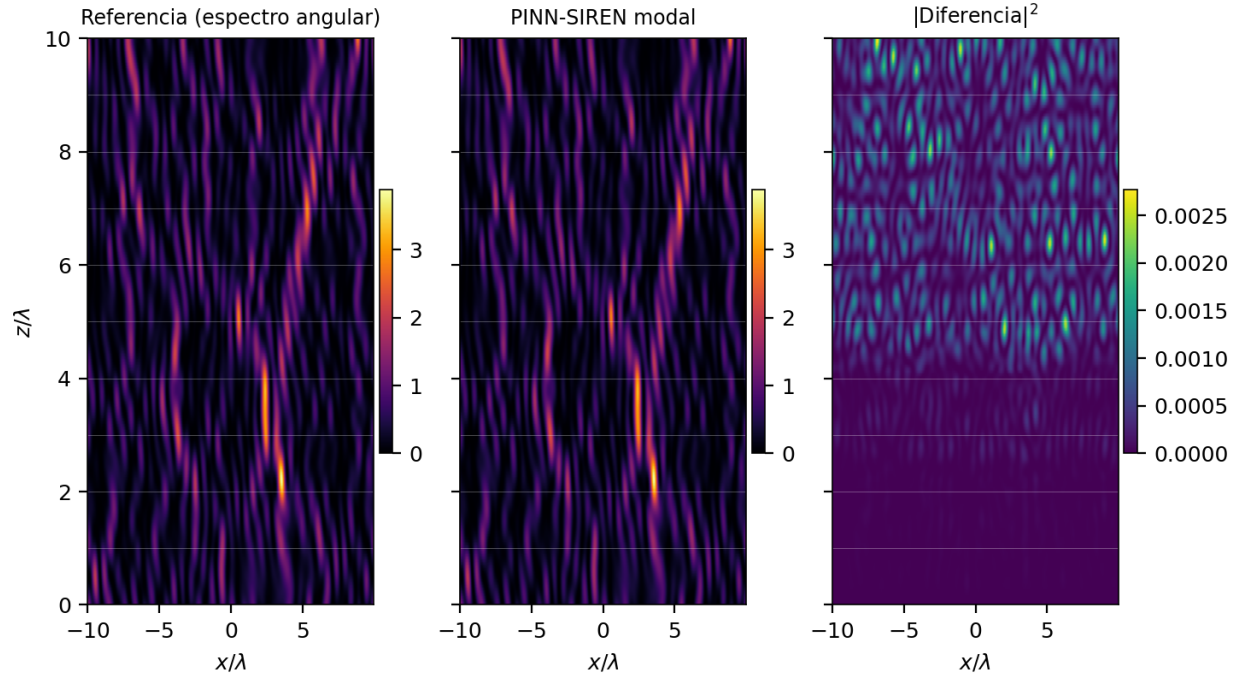
Figura 4.8. Mapas de intensidad |E|^2 sobre el plano de propagación completo (\tilde{x}, \tilde{z}) para la pantalla 42, con 0 \leq z \leq 10\lambda y -10 \leq \tilde{x} \leq 10 . Izquierda, la referencia por espectro angular restringida al subespacio propagante; centro, la PINN-SIREN modal, en la misma escala de color; derecha, el módulo al cuadrado de su diferencia, en escala propia. Las líneas horizontales tenues marcan las nueve interfaces entre los diez bloques de 1\lambda . Los dos primeros paneles son indistinguibles a simple vista: el pico de la diferencia vale 2.77 \times 10^{-3} frente a una intensidad máxima de 3.88, esto es, el 0.07% del pico. El tercer panel muestra dónde reside ese error, y es su información propia: la discrepancia es despreciable por debajo de z \approx 3\lambda y crece de forma visible a partir del quinto bloque, que es justamente donde empiezan las redes entrenadas en esta extensión y donde se acumula lo transferido por las anteriores. La presentación sigue el formato de sección transversal a lo largo de la propagación empleado por Hernández Nolasco (2003). Generada por scripts/build/figuras_nb03d_z10.py a partir de results/nb03_distance_pilot/z10_screen42_net42_adaptive_slabs_v1/adaptive_slabs_z10.npz .
