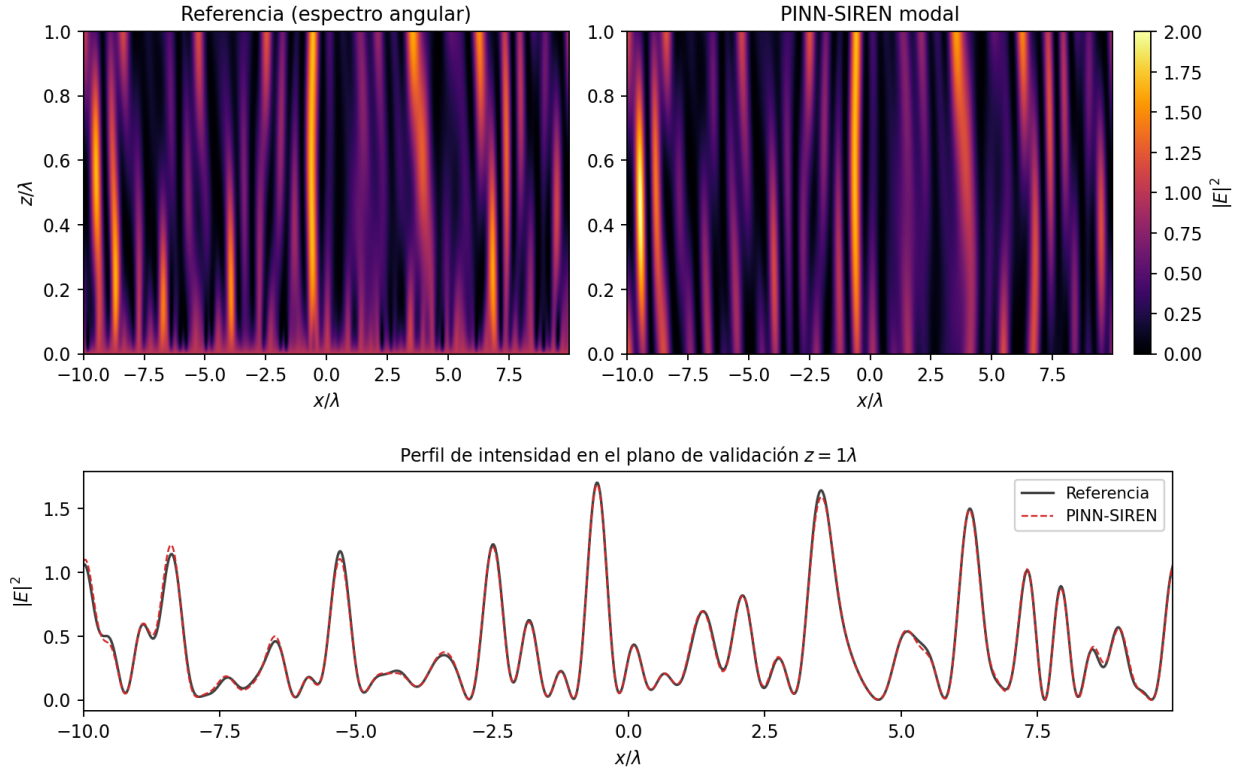
Figura 4.6. Patrón de speckle simulado, pantalla 42. Arriba, mapas de intensidad |E|^2 sobre el plano de propagación (\tilde{x}, \tilde{z}) para la referencia por espectro angular (izquierda) y para la PINN-SIREN modal (derecha), en la misma escala de color; la línea discontinua marca el plano de validación z = 1\lambda . Abajo, perfil transversal de intensidad en ese plano para ambas. La diferencia visible se concentra en las proximidades de \tilde{z} = 0 , donde la referencia presenta una estructura transversal fina que el modelo no reproduce y que se atenúa al propagar: es la contribución evanescente cuantificada en §4.4.9, irrepresentable por una base truncada al cono propagante. En el plano de validación los dos perfiles se superponen, con L^2 = 3.819\% de campo complejo y contrastes de 0.9063 y 0.9012. Generada por scripts/experiments/nb03_figura_speckle.py a partir del modelo results/models/nb03_modal_pinn_siren_z1_screen42_omega1_finetune.pt y de la referencia results/nb03_angular_spectrum_reference_z1_corr0.10.npz .
