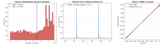
Fig. 2. Métricas adicionales de entrenamiento NB01. Panel A: distribución del error absoluto |\hat{E}(x) - E_{\text{exacta}}(x)| . Panel B: error relativo puntual (%). Panel C: dispersión de la predicción PINN contra la solución exacta, con la línea y = x como referencia de ajuste perfecto.
