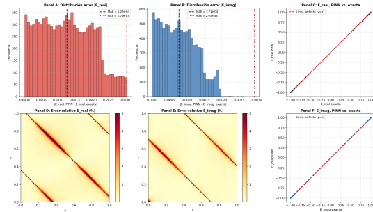
Fig. 4. Métricas adicionales de entrenamiento NB02. Paneles A-B: distribución del error absoluto |E_{\text{real}} - \hat{E}_{\text{real}}| y |E_{\text{imag}} - \hat{E}_{\text{imag}}| . Paneles C, F: dispersión de la predicción PINN contra la solución exacta para cada componente. Paneles D-E: error relativo puntual (%) en la malla 100 \times 100 ; los valores más altos se concentran en bandas antidiagonales ( x + y \approx \text{const.} ) donde la solución exacta cruza por cero, no en las esquinas del dominio. La curva de pérdida de entrenamiento se muestra en el Panel C3 de la Figura 3.
