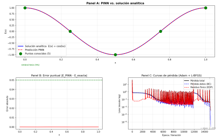
Fig. 1. Validación PINN-SIREN para Helmholtz 1D. Panel A: comparación entre la predicción de la red y la solución analítica E_{\text{exacta}}(x) = \cos(kx) en 1,000 puntos uniformes en [0, 1] . Panel B: error puntual |\hat{E}(x) - E_{\text{exacta}}(x)| . Panel C: curva de pérdida total durante las fases Adam y L-BFGS. Error L^2 = 0,006 \% , R^2 = 1,000000 . GPU: NVIDIA RTX 5050, SEED = 42.
