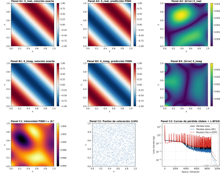
Fig. 3. Validación PINN-SIREN para Helmholtz 2D con campo complejo. Fila superior (A1-A3): solución analítica, predicción PINN-SIREN y error absoluto para E_{\text{real}} . Fila central (B1-B3): lo mismo para E_{\text{imag}} . Fila inferior: intensidad predicha I = |E|^2 (C1), puntos de colocación LHS (C2) y curvas de pérdida durante Adam y L-BFGS (C3). La diferencia visual entre solución exacta y predicción es indistinguible; los errores puntuales son del orden de 10^{-3} (ver Tabla 3). Malla de evaluación 100 \times 100 , SEED = 42.
