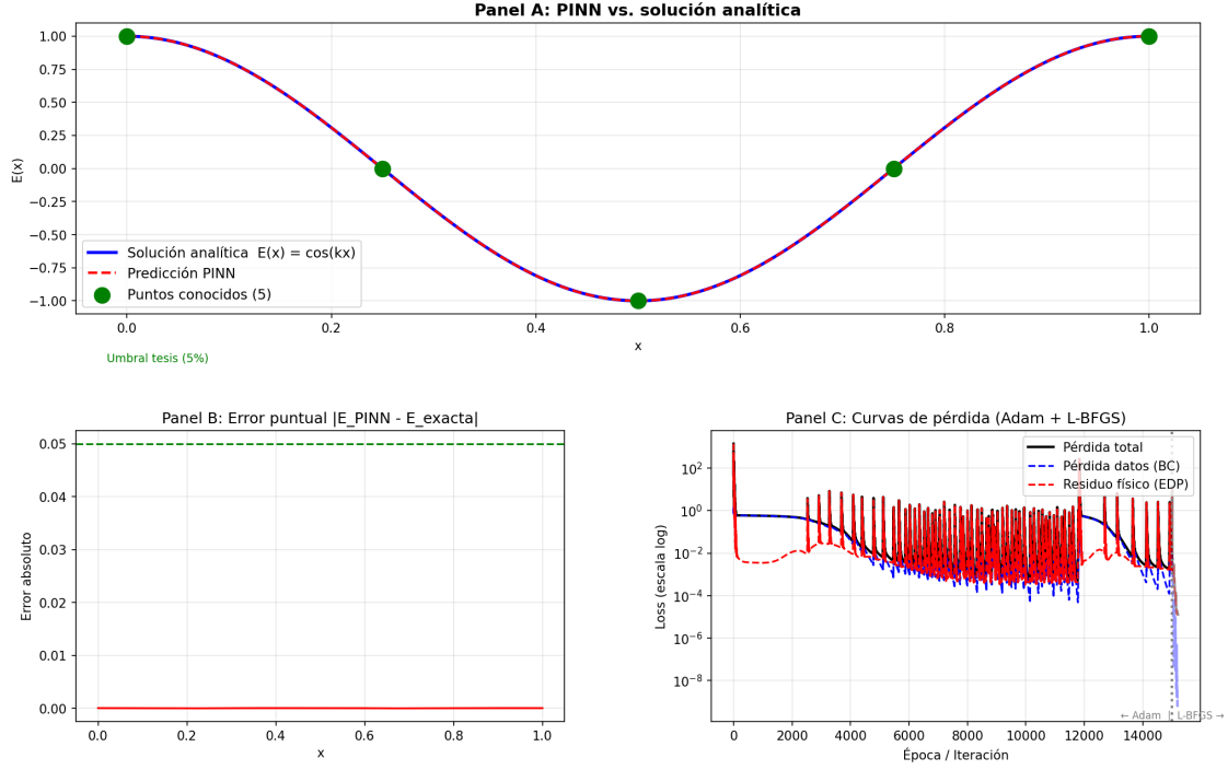
Figura 1: Validación PINN-SIREN para Helmholtz 1D. Panel A: comparación entre la predicción de la red y la solución analítica E_{exacta}(x) = \cos(kx) en 1,000 puntos uniformes en [0, 1] . Panel B: error puntual |\hat{E}(x) - E_{exacta}(x)| . Panel C: curva de pérdida total durante las fases Adam y L-BFGS. Error L^2 = 0,006 \% , R^2 = 1,000000 . GPU: NVIDIA RTX 5050, SEED = 42.
