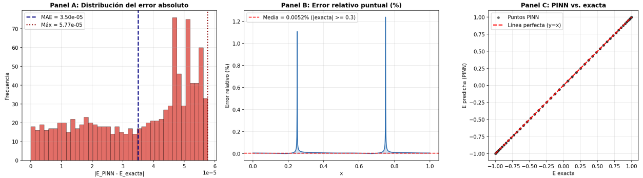
Figura 2: Métricas adicionales de entrenamiento NB01. Panel A: distribución del error absoluto |\hat{E}(x) - E_{exacta}(x)| . Panel B: error relativo puntual (%). Panel C: dispersión de la predicción PINN contra la solución exacta, con la línea y = x como referencia de ajuste perfecto.
