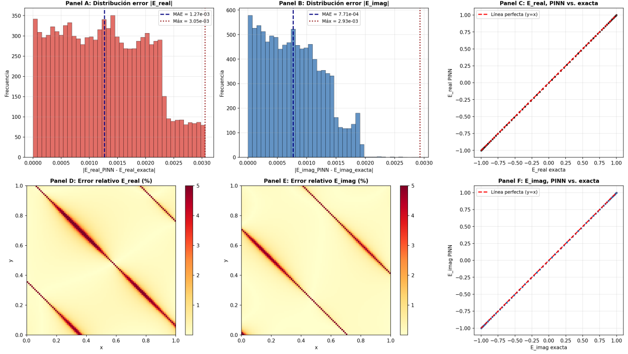
Figura 4: Métricas adicionales de entrenamiento NB02. Paneles A-B: distribución del error absoluto |E_{\text{real}} - \hat{E}_{\text{real}}| y |E_{\text{imag}} - \hat{E}_{\text{imag}}| . Paneles C, F: dispersión de la predicción PINN contra la solución exacta para cada componente. Paneles D-E: error relativo puntual (%) en la malla 100 \times 100 ; los valores más altos se concentran en bandas antidiagonales ( x + y \approx \text{const.} ) donde la solución exacta cruza por cero, no en las esquinas del dominio. La curva de pérdida de entrenamiento se muestra en el Panel C3 de la figura 3.
