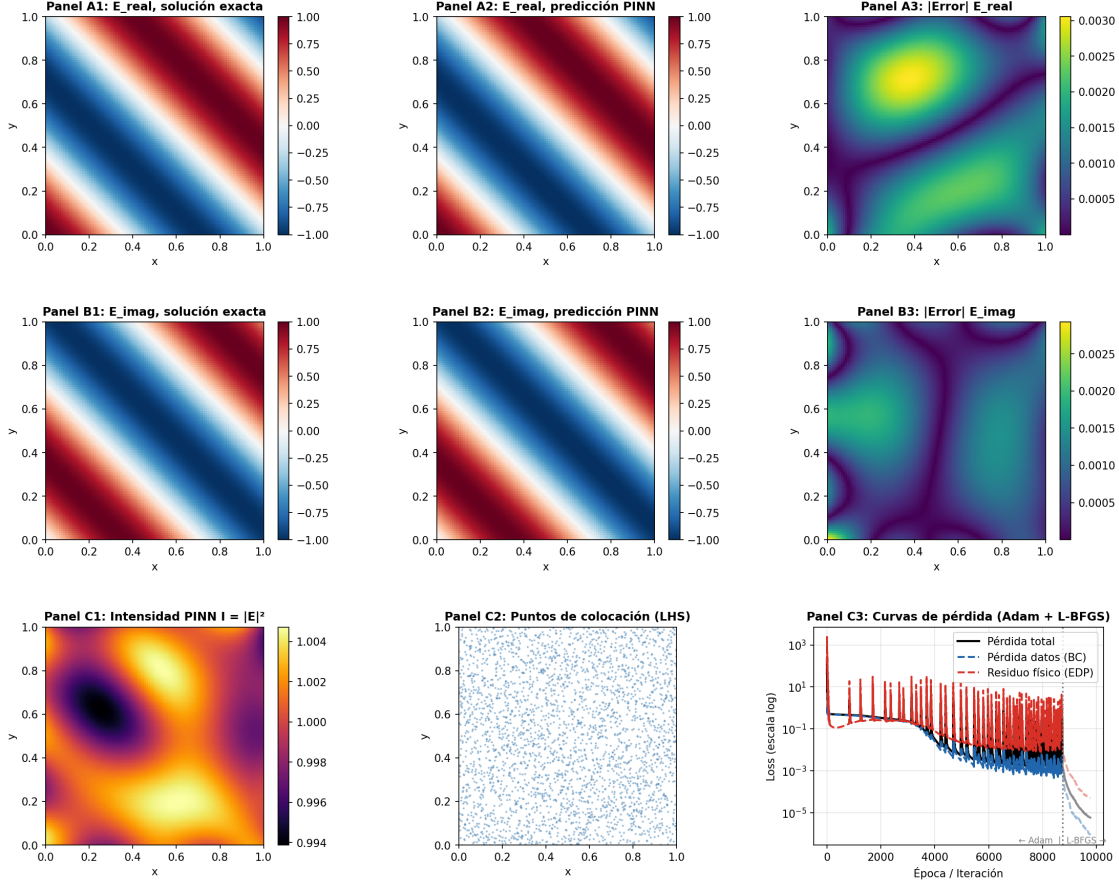
Figura 3: Validación PINN-SIREN para Helmholtz 2D con campo complejo. Fila superior (A1-A3): solución analítica, predicción PINN-SIREN y error absoluto para E_{\text{real}} . Fila central (B1-B3): lo mismo para E_{\text{imag}} . Fila inferior: intensidad predicha I = |E|^2 (C1), puntos de colocación LHS (C2) y curvas de pérdida durante Adam y L-BFGS (C3). La diferencia visual entre solución exacta y predicción es indistinguible; los errores puntuales son del orden de 10^{-3} (ver tabla 3). Malla de evaluación 100 \times 100 , SEED = 42.
