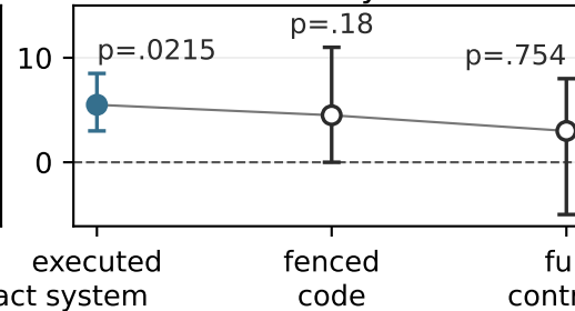
Llama · Python
