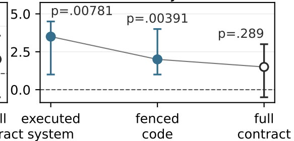
Llama · Java
