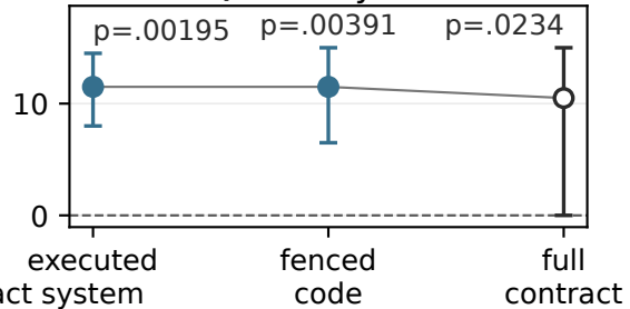
Qwen · Python
