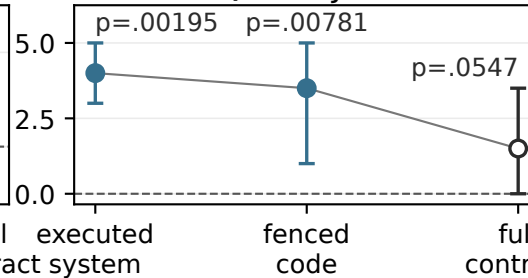
Qwen · Java
