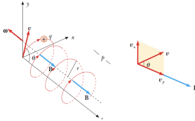
Figura 13.3: Moto elicoidale di una particella con carica positiva in campo magnetico uniforme
