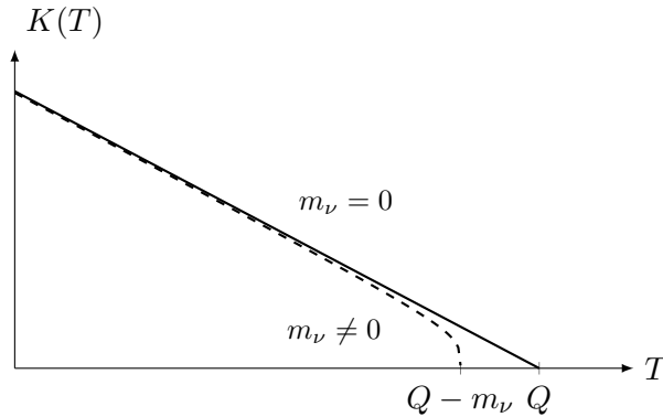
Figura II.2.: Diagramma di Kurie, con e senza massa del neutrino.
