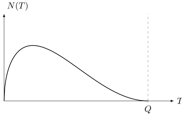
Figura II.1.: Spettro in energia degli elettroni emessi nel decadimento \beta .
