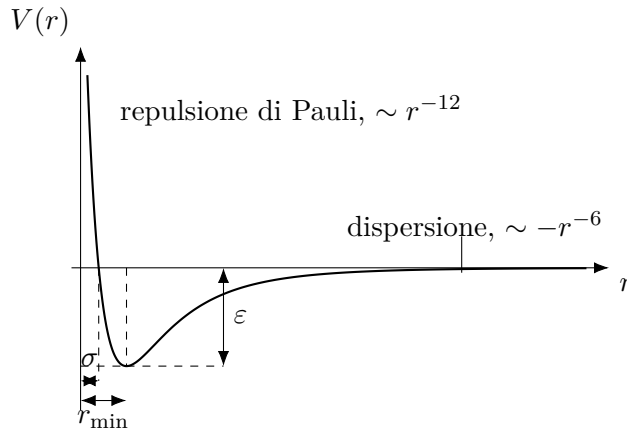
Figura 5.6: Potenziale di Lennard-Jones.
