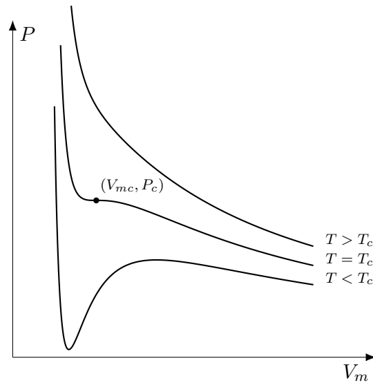
Figura 6.2: Isotherme di van der Waals.
