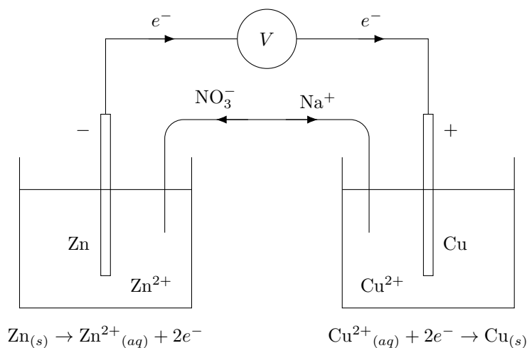
Figura 13.1: Schema della pila Daniell
