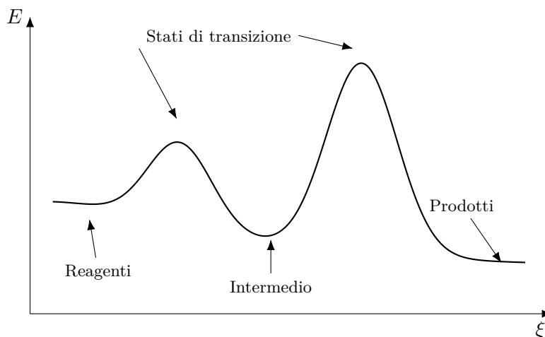
Figura 10.1: Profilo energetico di una reazione a due stadi.
