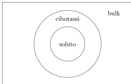
Figura 11.1: Struttura di una soluzione attorno a una molecola di soluto.
