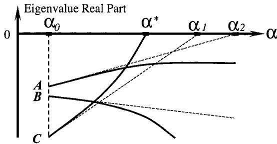
Figure 4.2. Eigenvalue real part vs. parameter \alpha .
