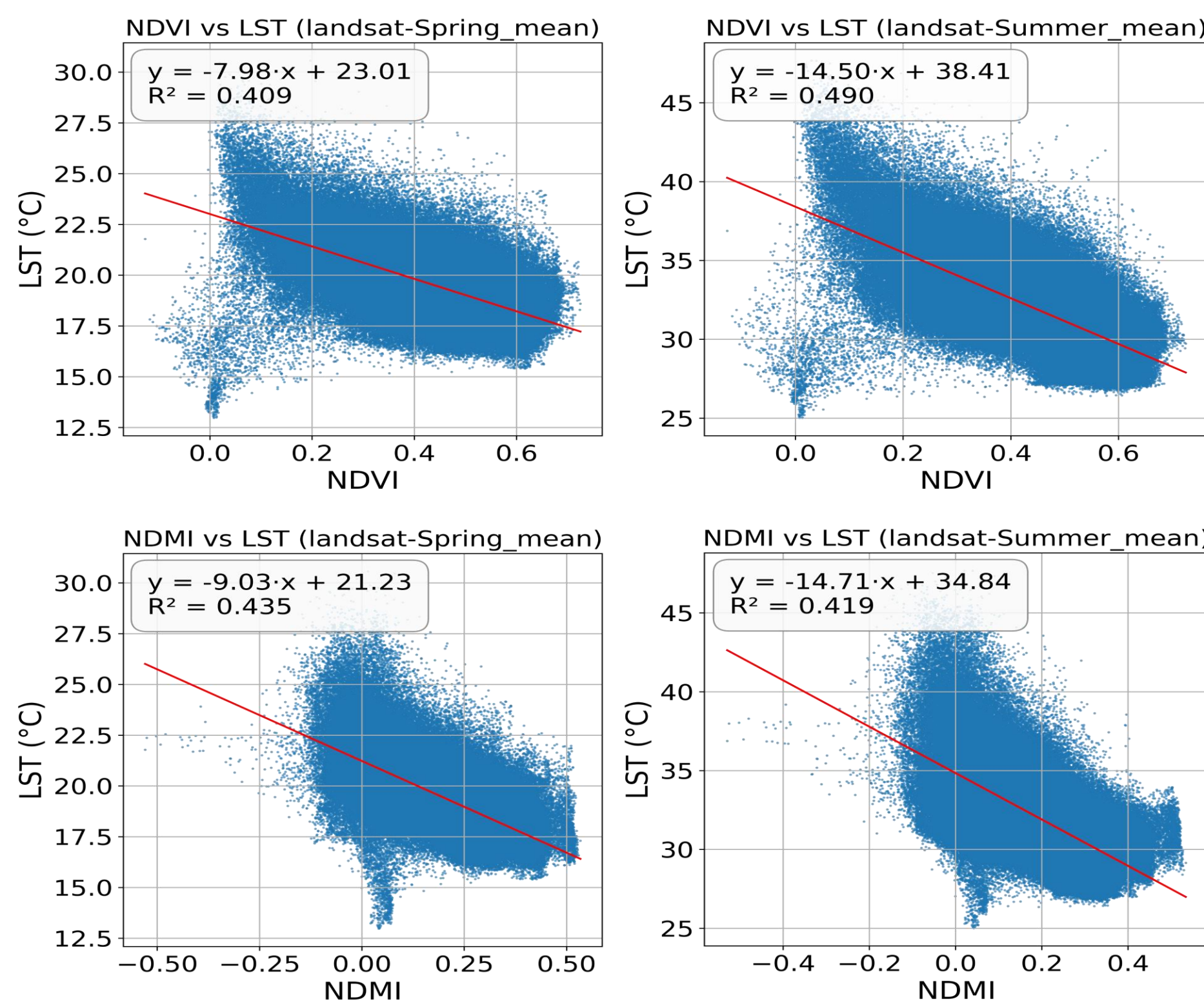
Abbildung 7: Korrelation zwischen LST und NDVI/NDMI
