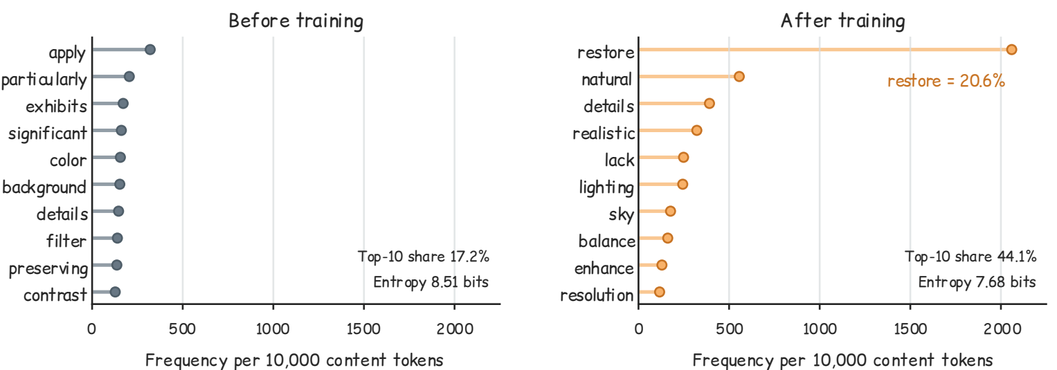
(d). Token Frequency Change
