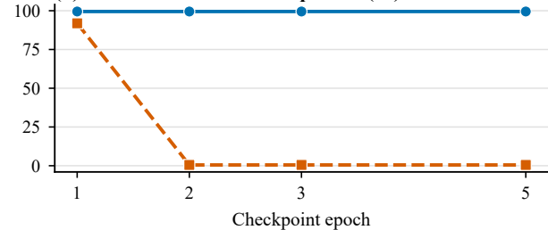
(d) Normalized-solution uniqueness (%)
