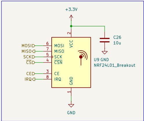
NRF24L01 Breakout
