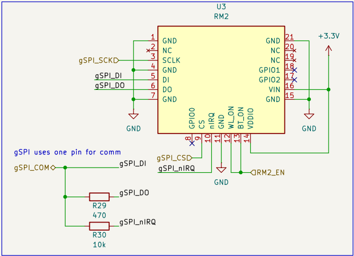
Radio Module 2
