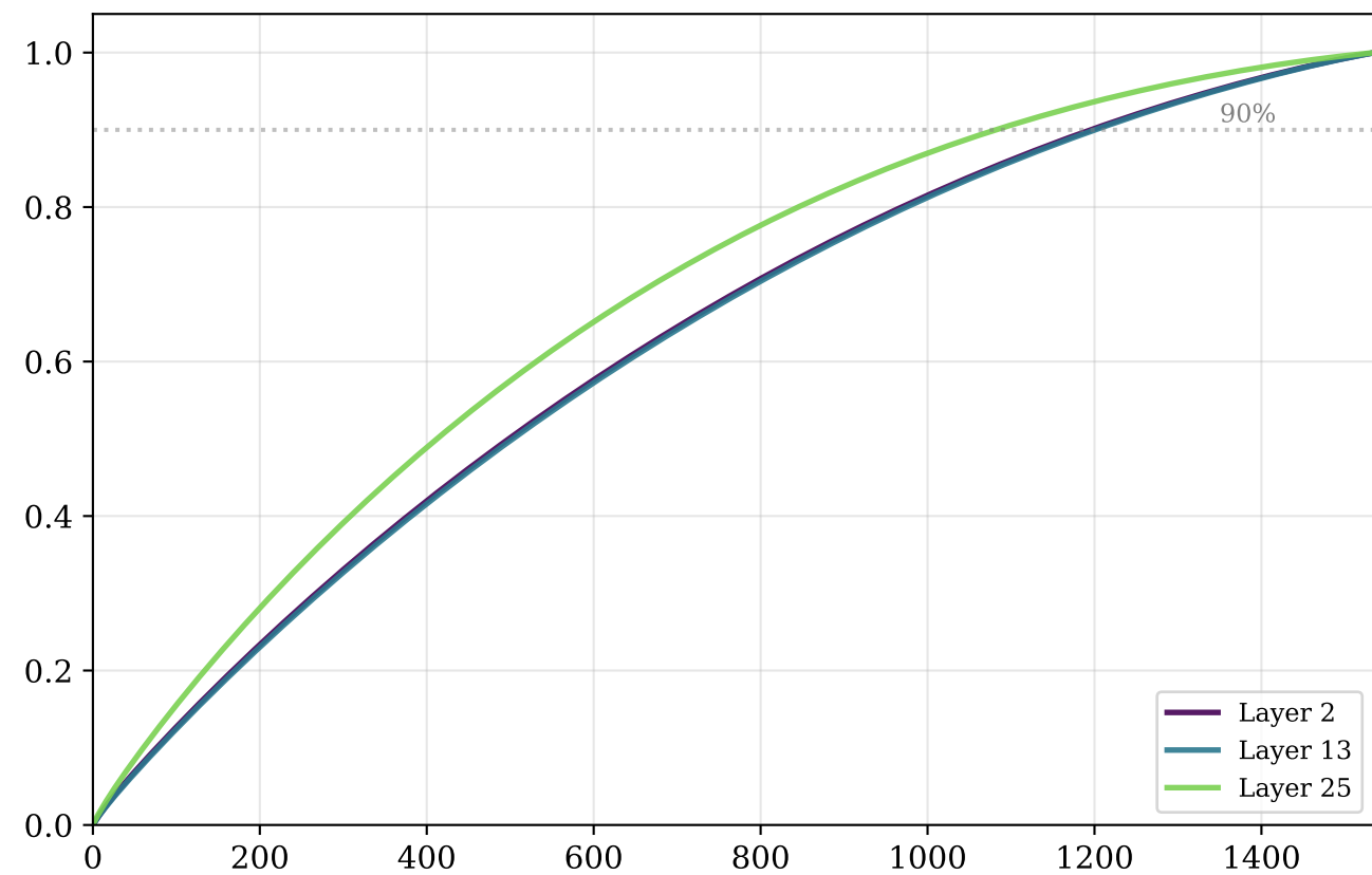
Muon + SFT
