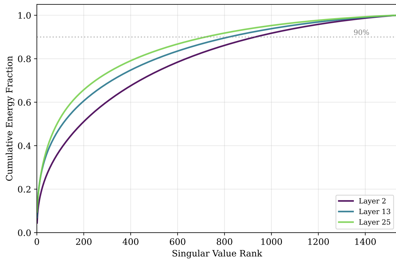
AdamW + SFT
