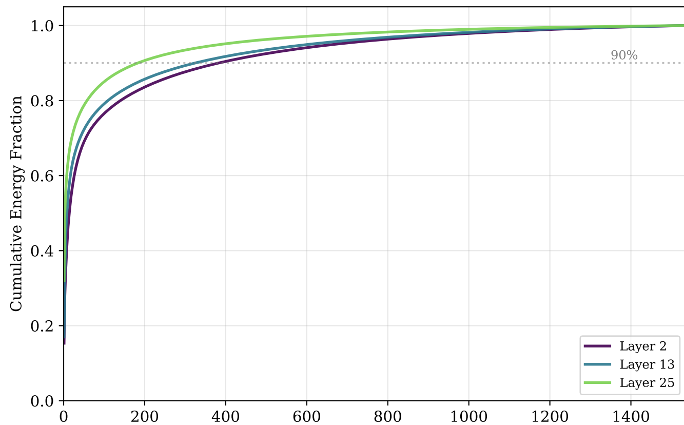
AdamW + SFT
