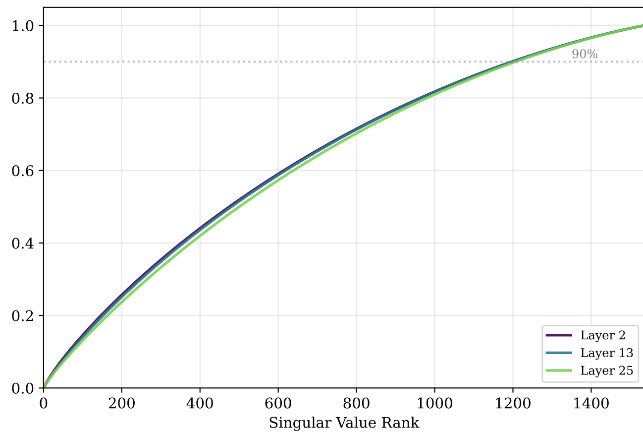
Muon + SFT
