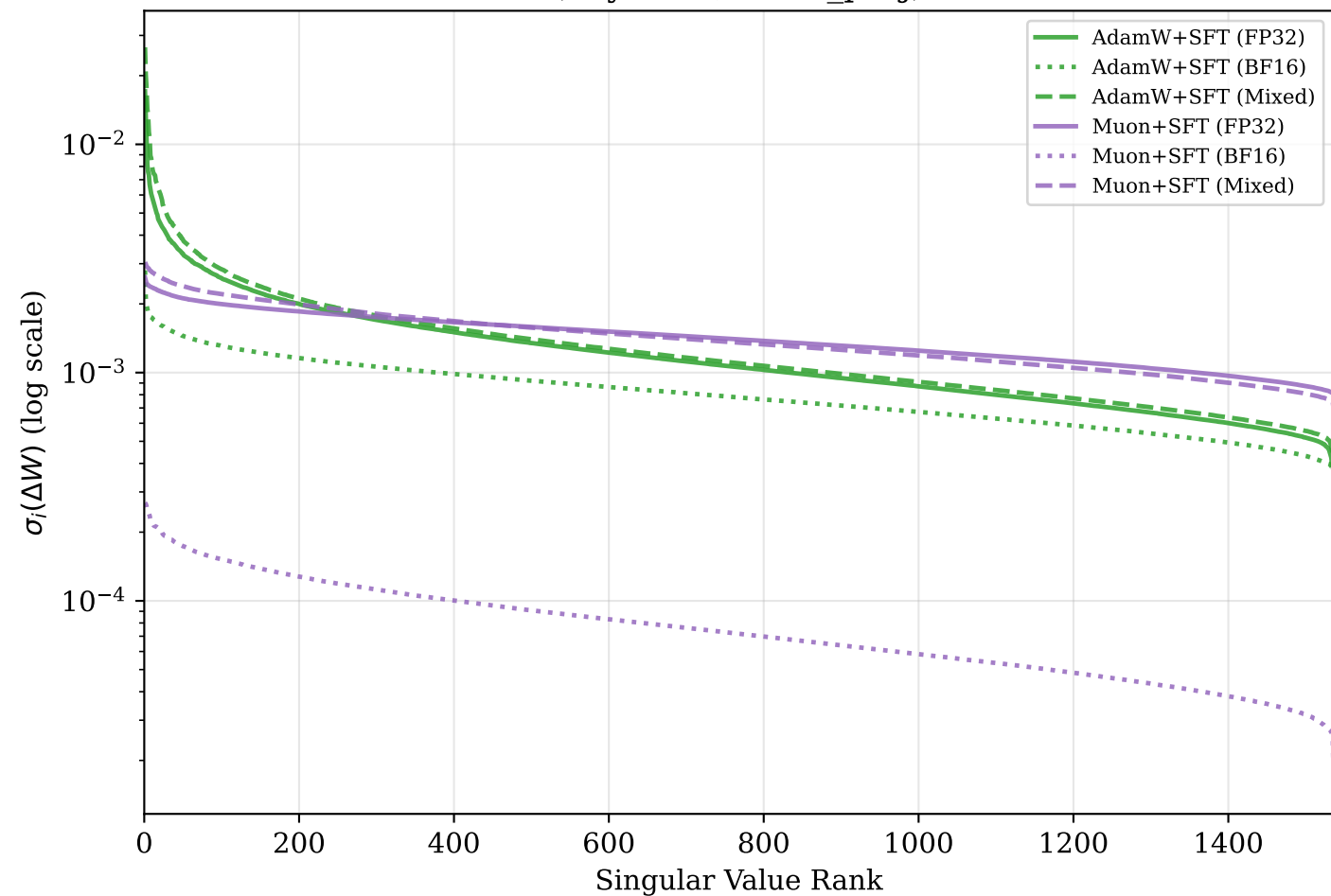
SFT: Raw SV Magnitudes (Layer 13, down_proj)
