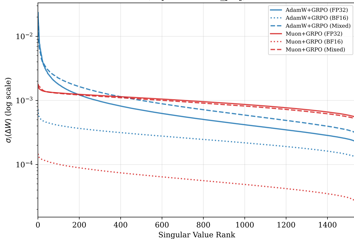
GRPO: Raw SV Magnitudes (Layer 13, down_proj)
