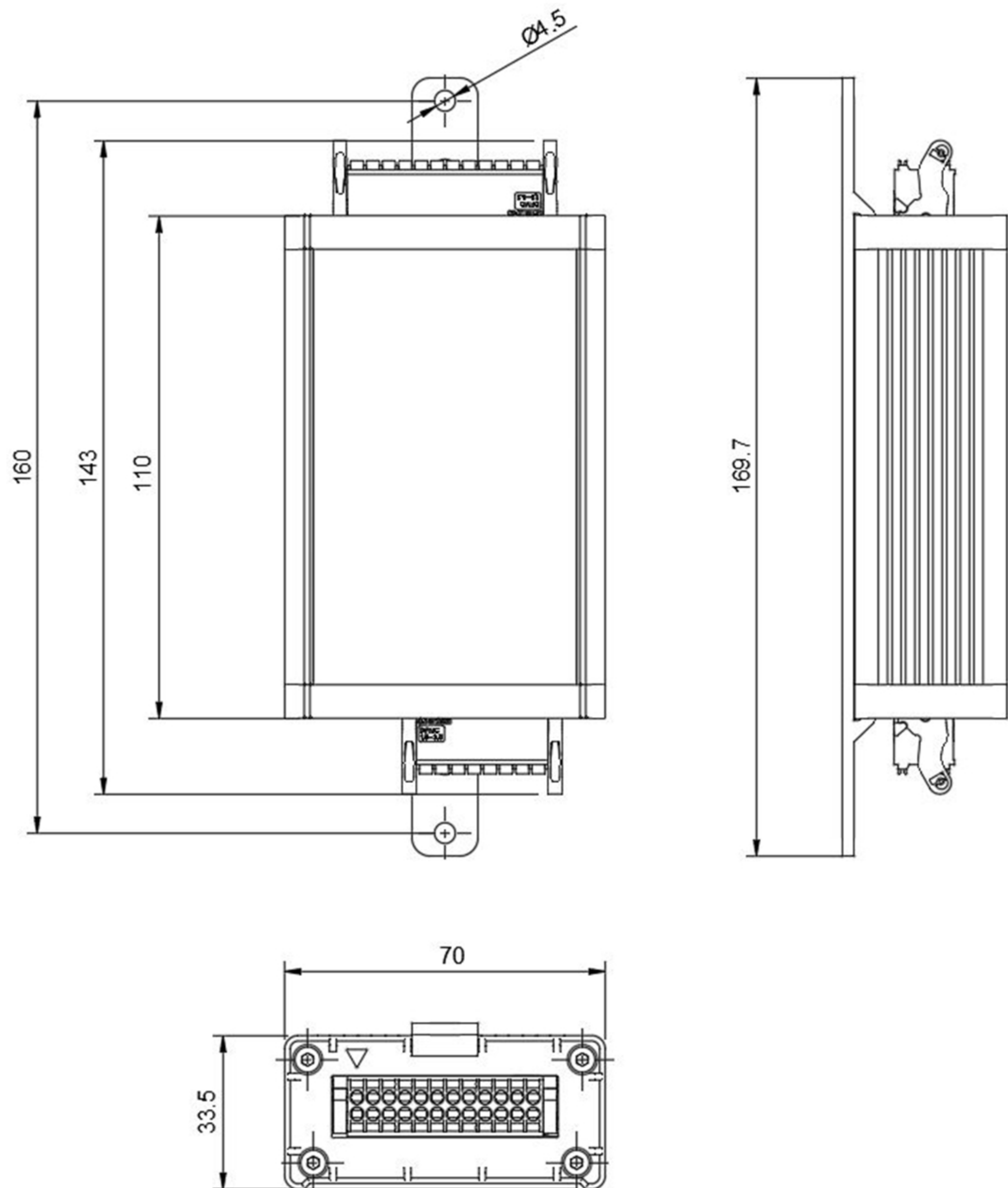
BareMetal PLC M с креплением на поверхность
