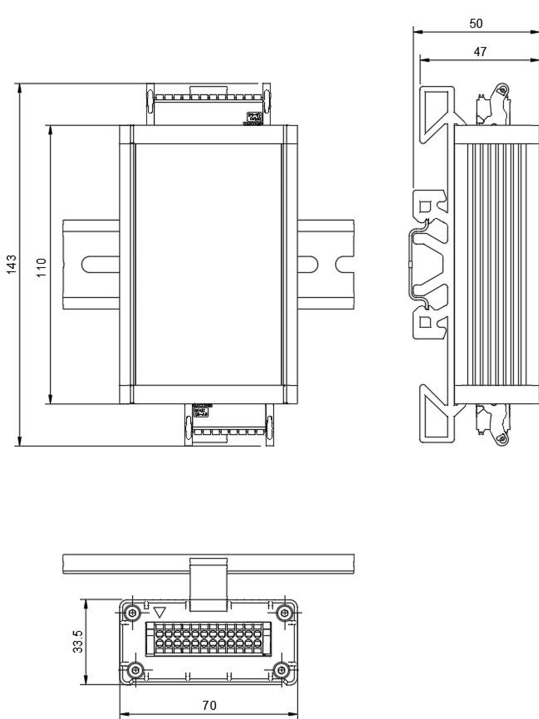
BareMetal PLC M с креплением на DIN рейку
