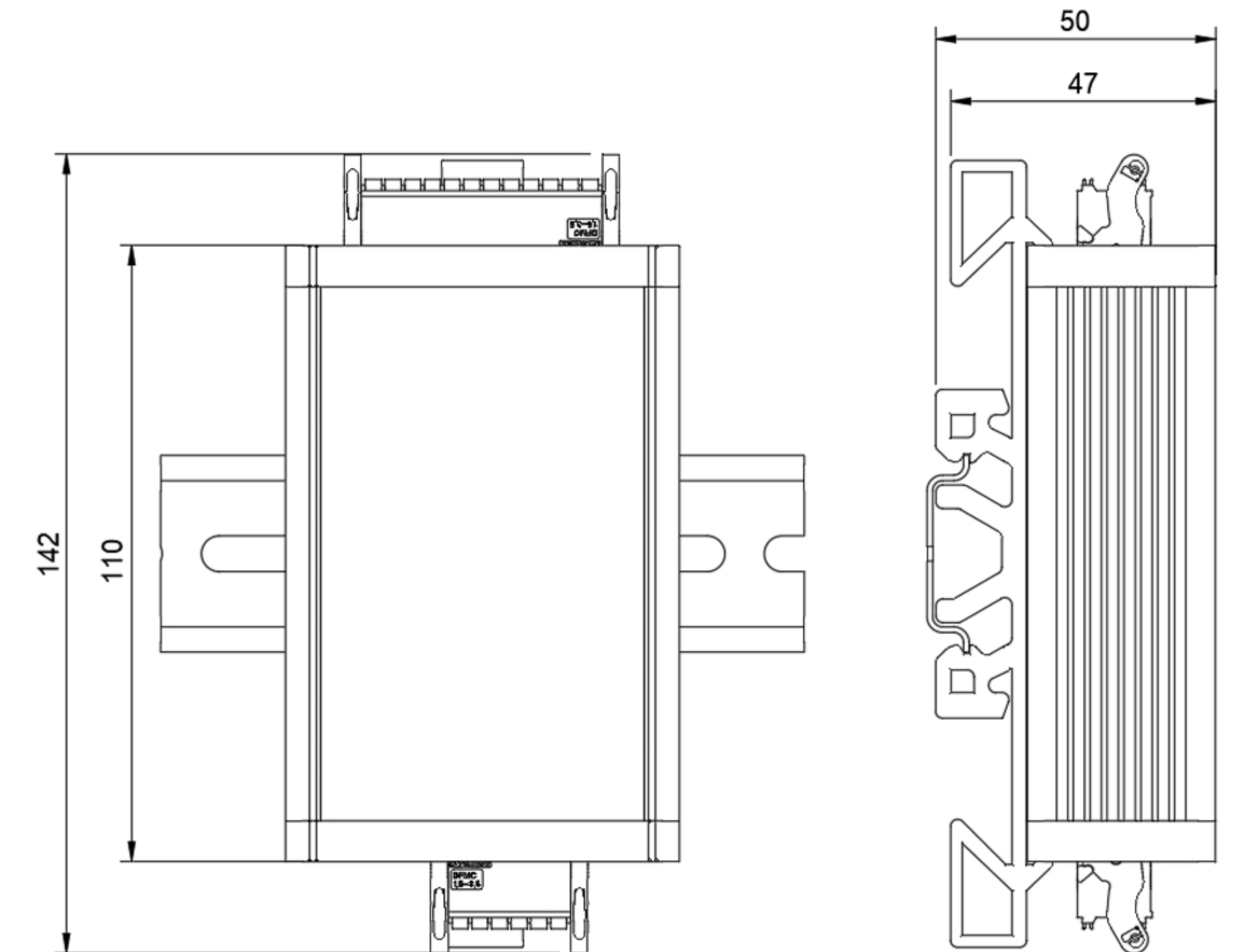
BareMetal PLC XL с креплением на DIN рейку
