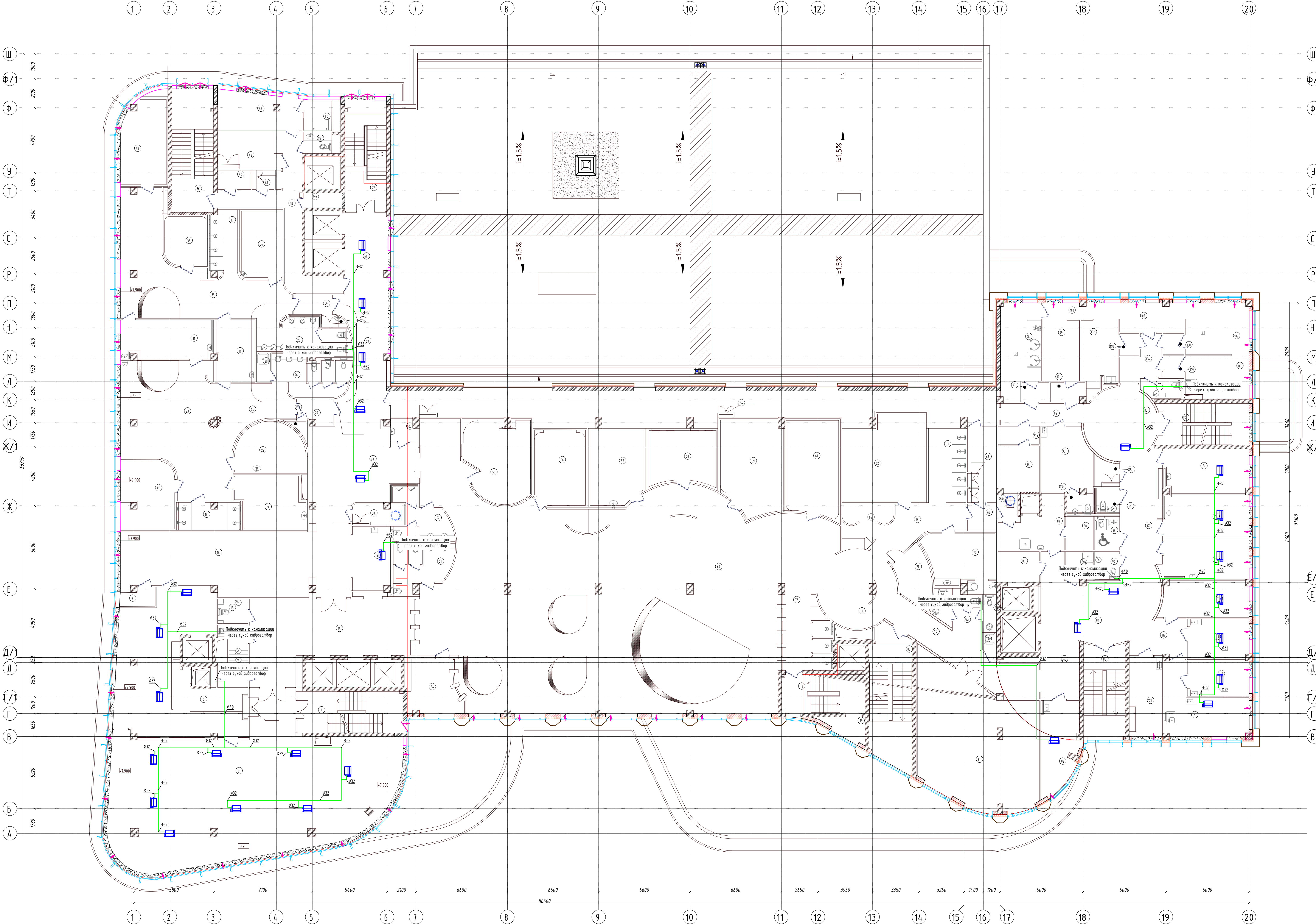
План системы дренажа кондиционирование 2-го этажа на отм. +7,350
