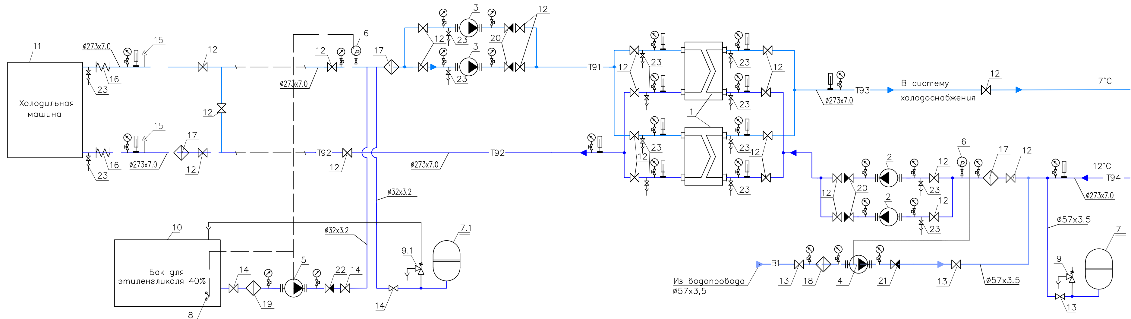
Принципиальная схема
