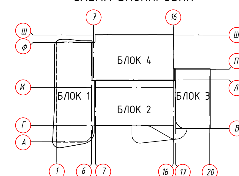
СХЕМА БЛОКИРОВКИ
