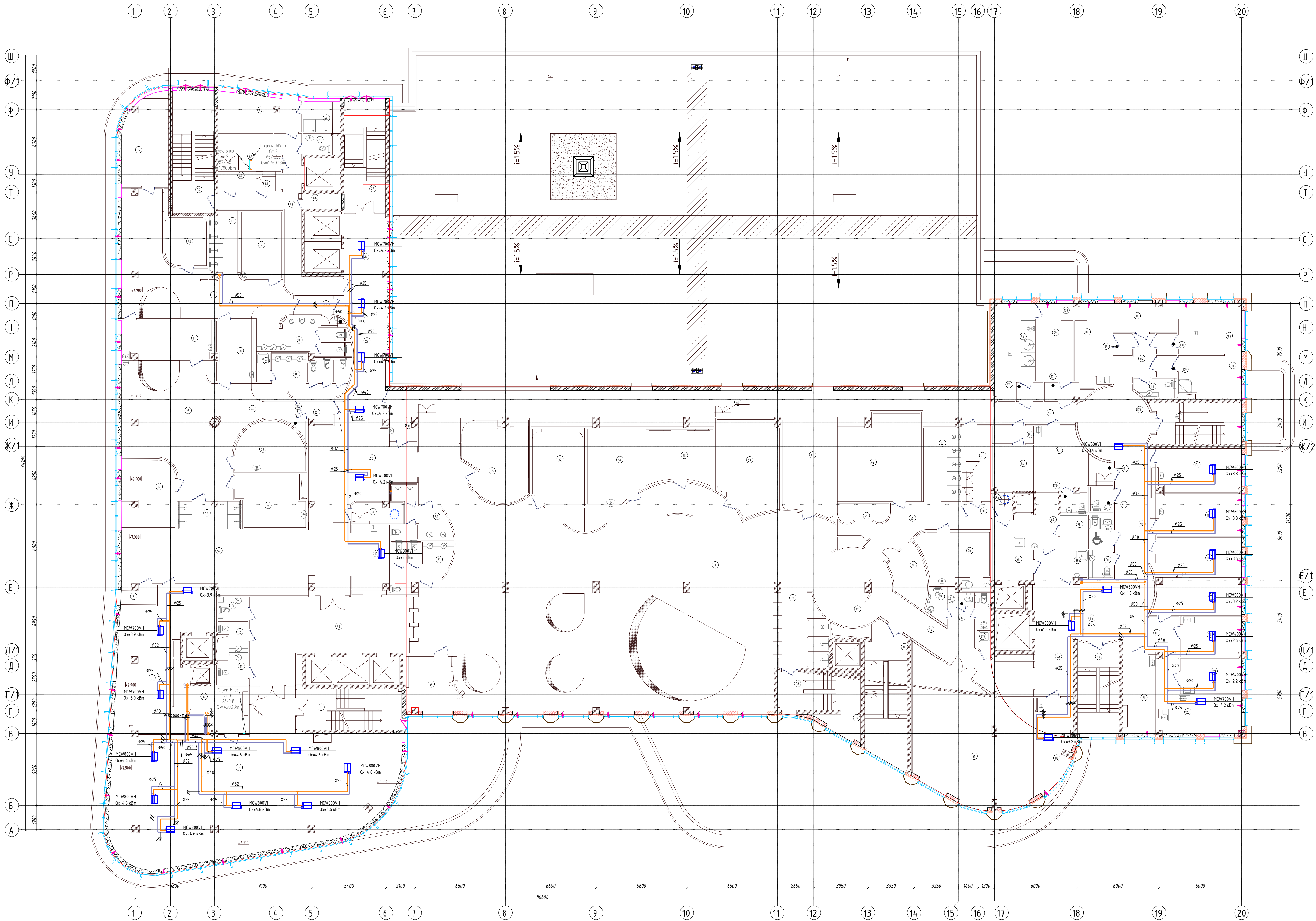
План кондиционирование 2-го этажа на отм. +7,350
