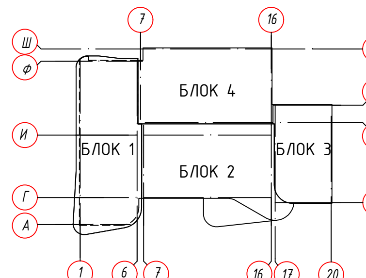
СХЕМА БЛОКИРОВКИ
