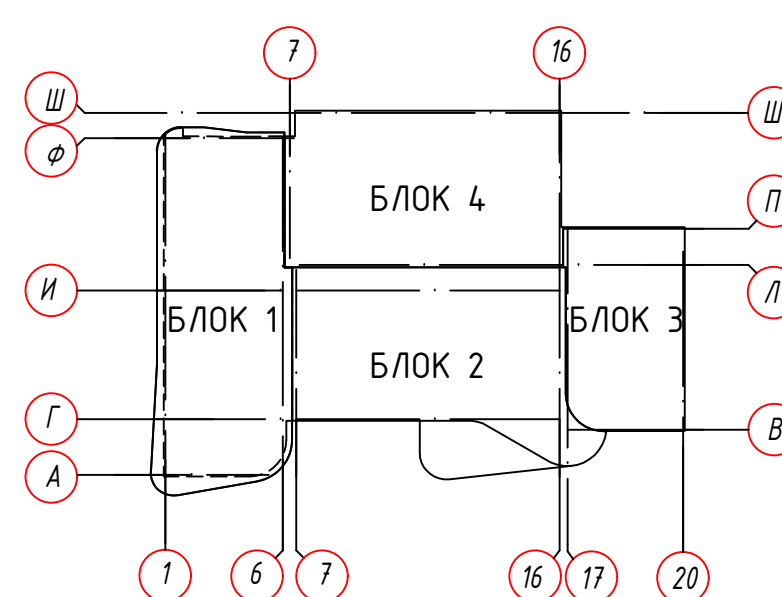
СХЕМА БЛОКИРОВКИ
