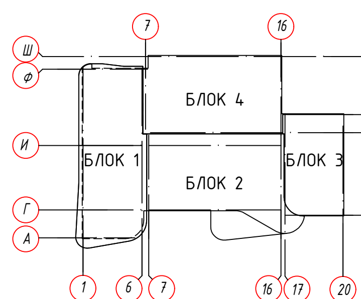
СХЕМА БЛОКИРОВКИ
