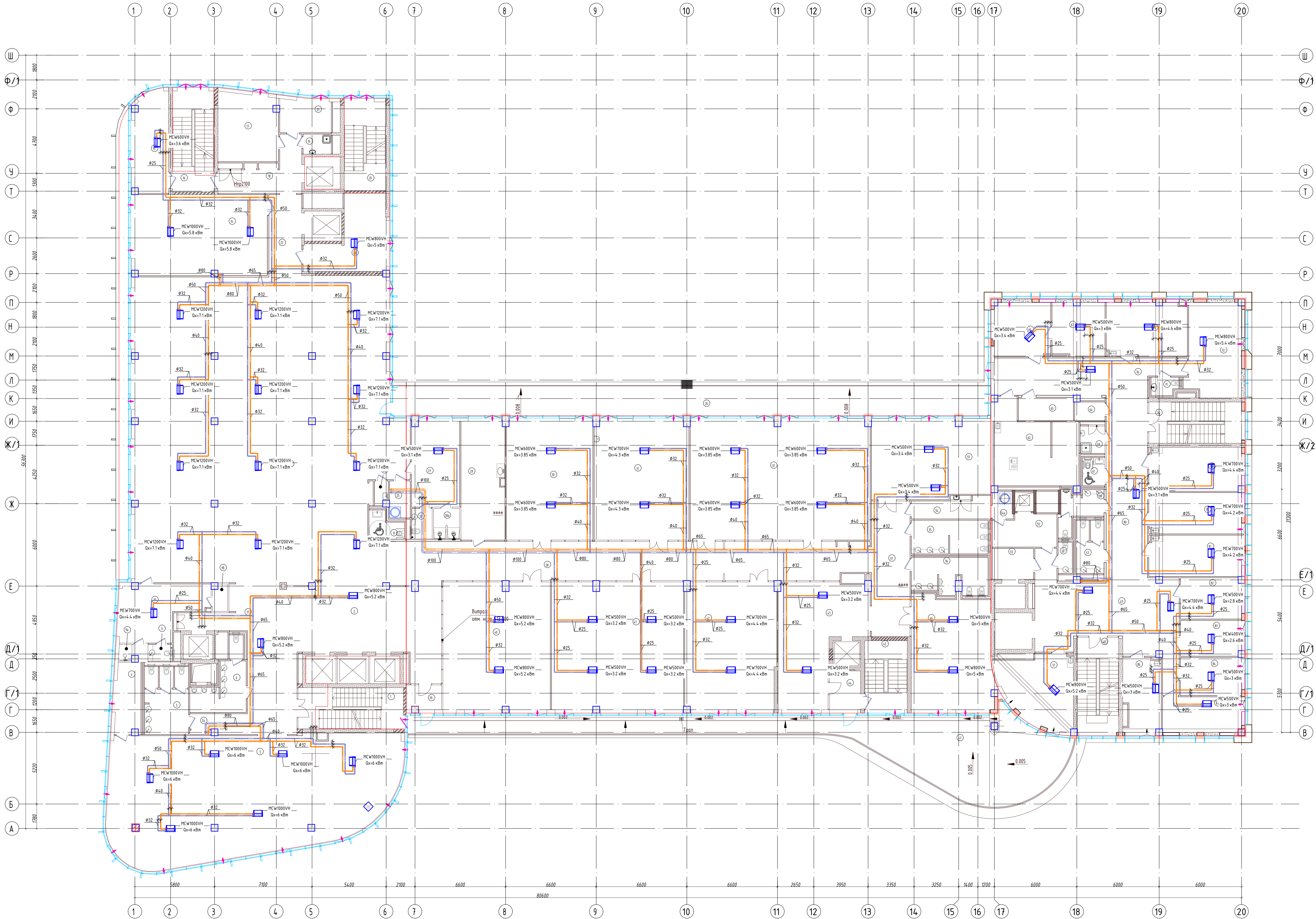
План 3 этажа
