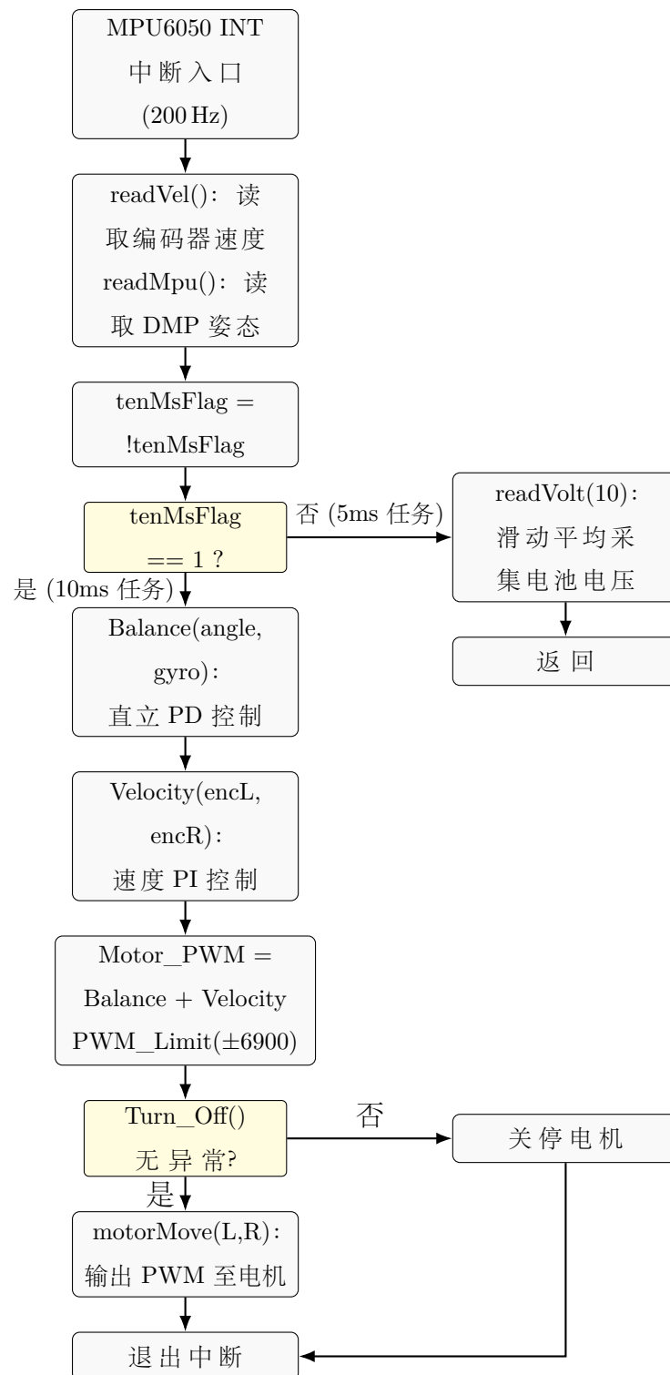
图 3.3 MPU6050 外部中断 ISR 执行流程图
