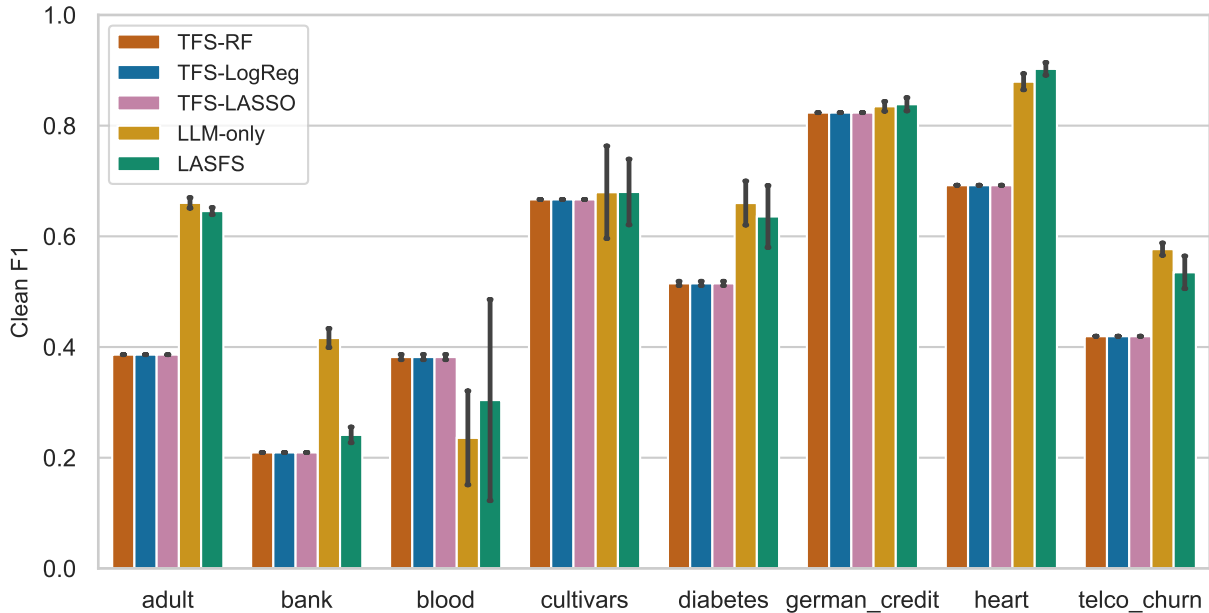
Clean Deployment F1
