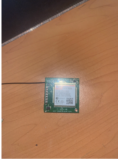
Figura 4: Módulo A7670SA utilizado durante la etapa actual de desarrollo.
