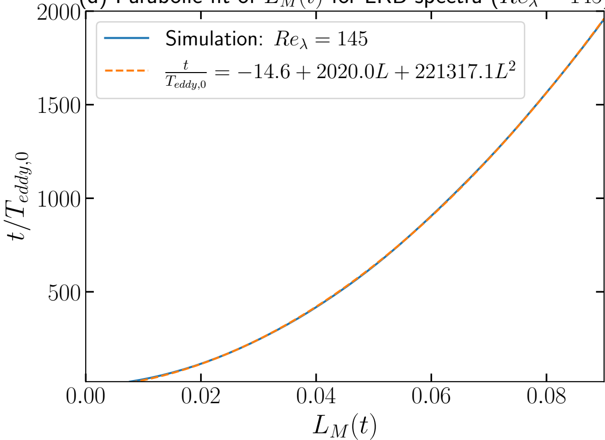
(d) Parabolic fit of L_M(t) for LKB spectra ( Re_\lambda = 145 )
