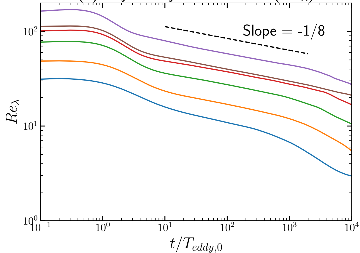
(d) Taylor Reynolds number ( Re_\lambda )
