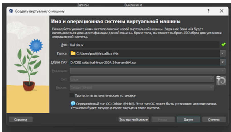
Рисунок 2.1: Создание ВМ
