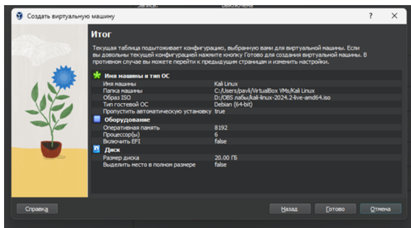
Рисунок 2.2: Запуск ВМ
