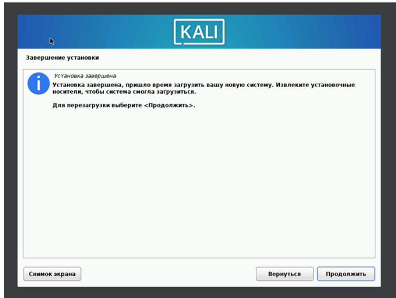
Рисунок 2.5: Перезагрузка системы
