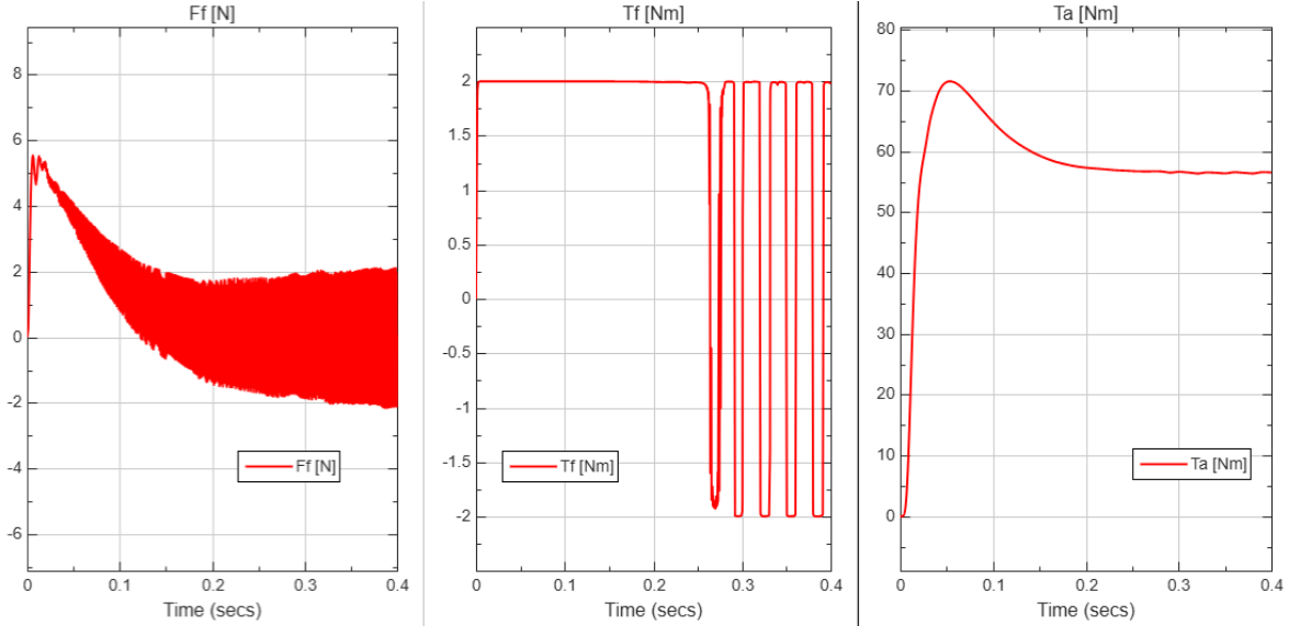
Figura 17: Perturbaciones F_f , T_f y T_a durante la respuesta a referencia trapezoidal de 5^\circ
