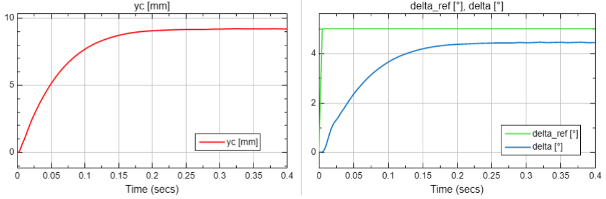
Figura 18: Respuesta \delta(t) y y_c(t) ante una referencia trapezoidal de 5^\circ
