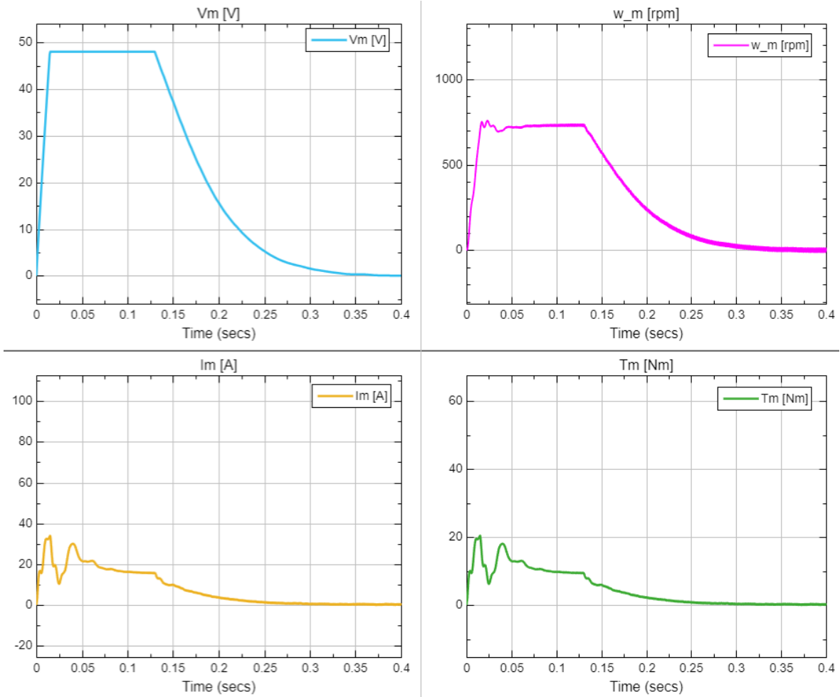
Figura 14: Variables eléctricas y mecánicas del motor ante referencia trapezoidal de 35^\circ
