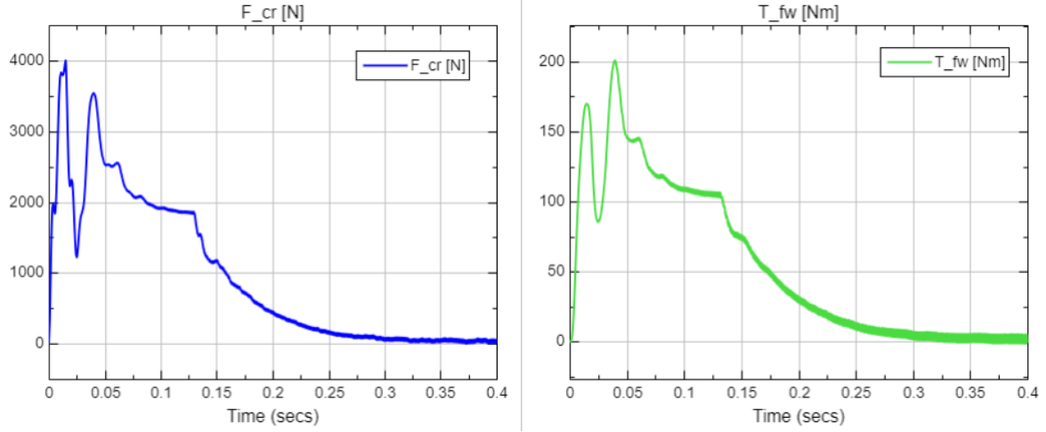
Figura 16: Fuerza F_{cr} y torque T_{fw} efectivos aplicados sobre cremallera y rueda, respectivamente.
