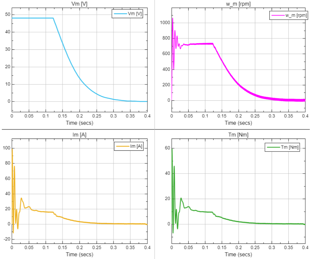
Figura 12: Parámetros del motor ante entrada escalón de 35^\circ
