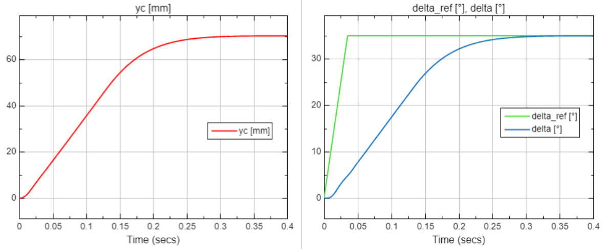
Figura 13: Respuesta \delta(t) y y_c(t) ante una referencia trapezoidal de 35^\circ
