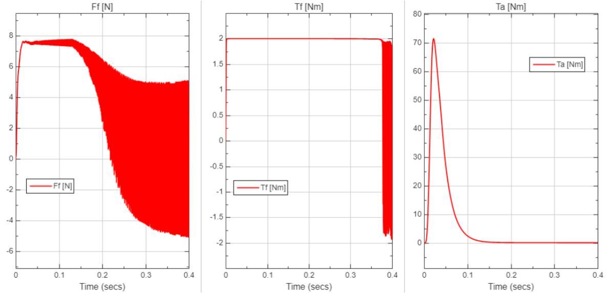
Figura 15: Perturbaciones F_f , T_f y T_a durante la respuesta a referencia trapezoidal de 35°
