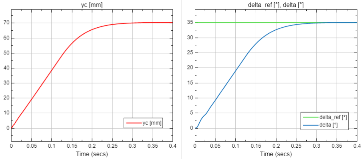
Figura 11: Respuesta \delta(t) y y_c(t) ante una referencia escalón de 35^\circ
