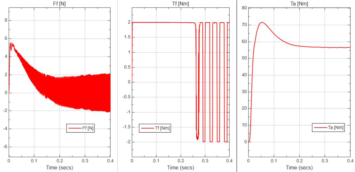
Figura 17: Perturbaciones F_f , T_f y T_a durante la respuesta a referencia trapezoidal de 5^\circ
