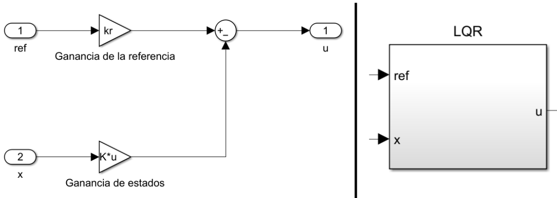
Figura 7: Bloque de controlador LQR en Simulink
