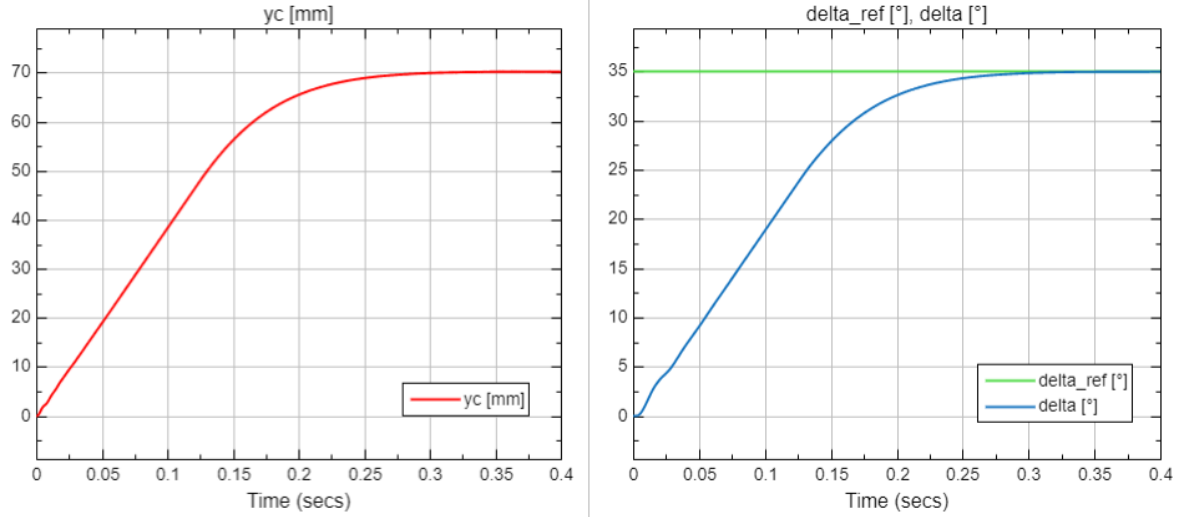
Figura 12: Respuesta \delta(t) y y_c(t) ante una referencia escalón de 35^\circ
