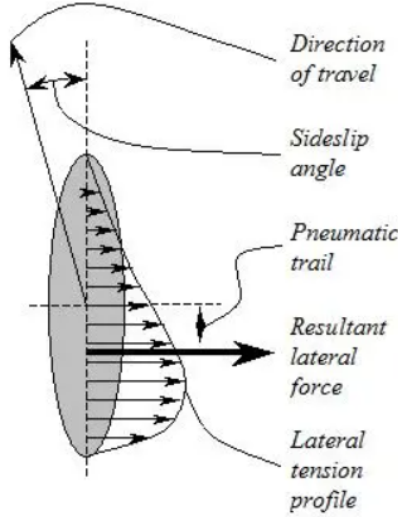
Figura 11: Fuerza resultante lateral debido a una rotación de la rueda en sentido horario
