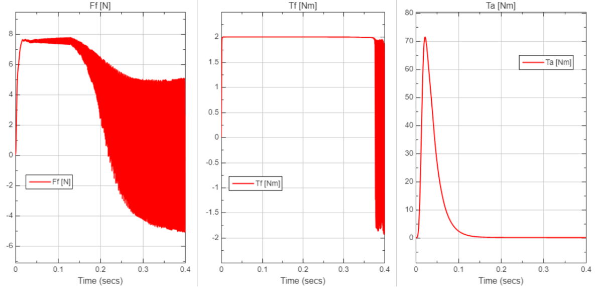
Figura 16: Perturbaciones F_f , T_f y T_a durante la respuesta a referencia trapezoidal de 35°
