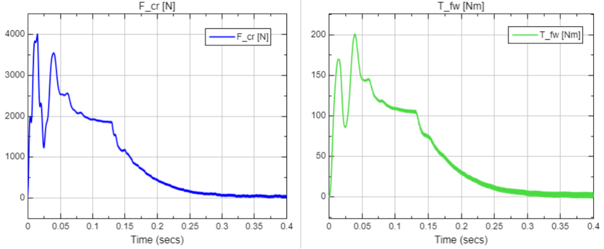
Figura 17: Fuerza F_{cr} y torque T_{fw} efectivos aplicados sobre cremallera y rueda, respectivamente.
