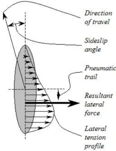
Figura 7: Fuerza resultante lateral debido a una rotación de la rueda en sentido horario
