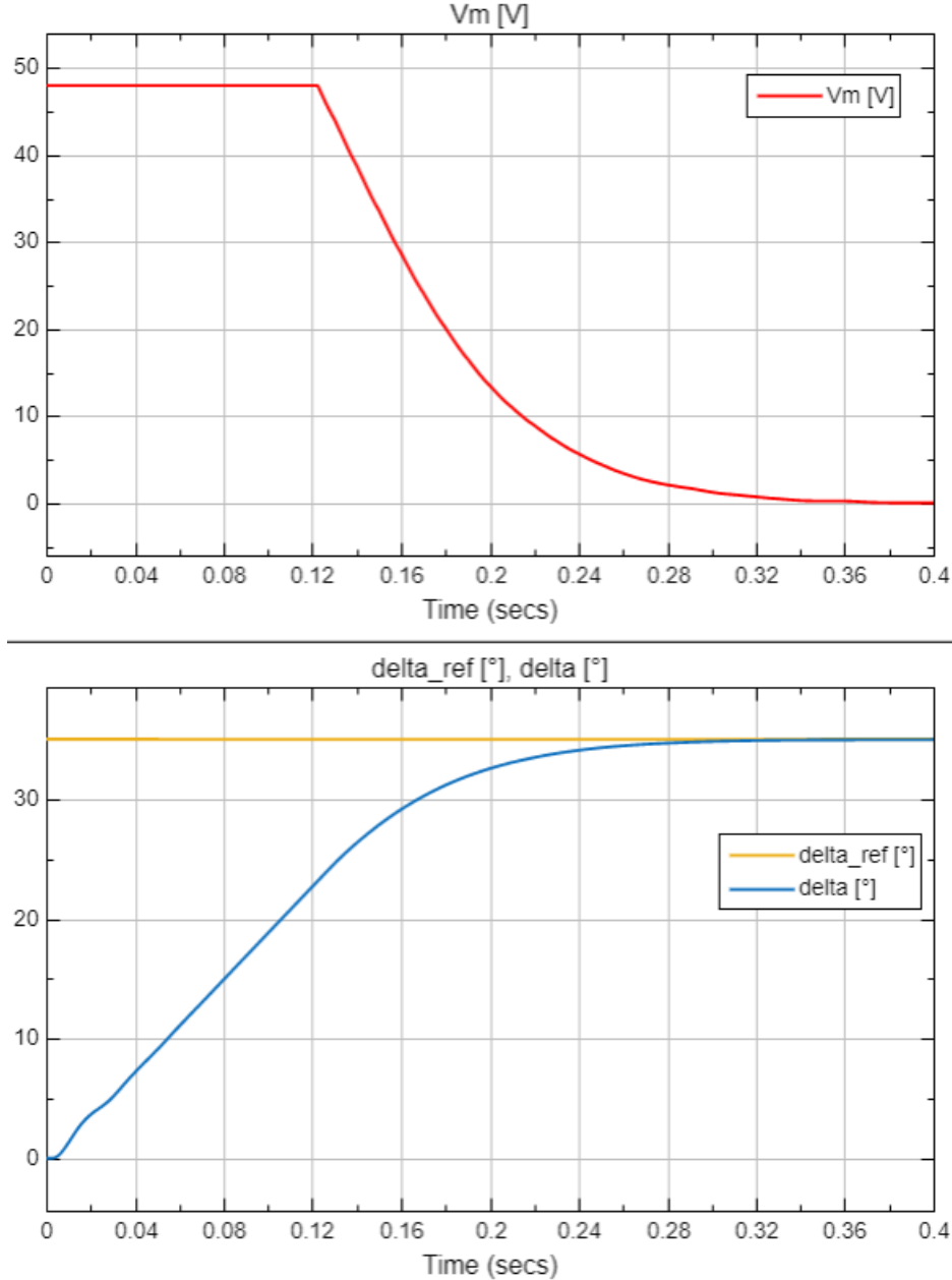
Figura 8: Respuesta del ángulo de las ruedas \delta(t) ante una referencia escalón de 35^\circ
