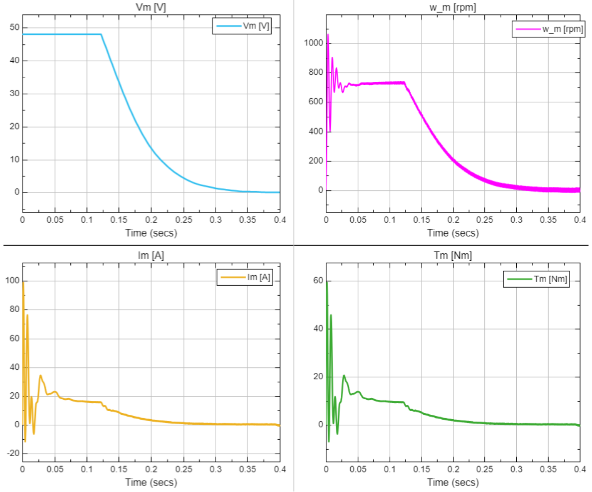
Figura 13: Parámetros del motor ante entrada escalón de 35^\circ
