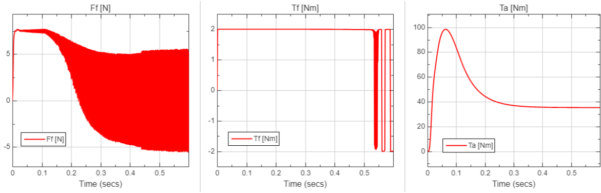
Figura 15: Perturbaciones F_f , T_f y T_a durante la respuesta a referencia trapezoidal de 35^\circ
