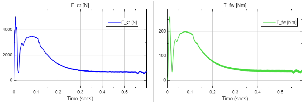
Figura 16: Fuerza F_{cr} y torque T_{fw} efectivos aplicados sobre cremallera y rueda, respectivamente.
