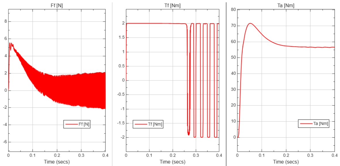
Figura 18: Perturbaciones F_f , T_f y T_a durante la respuesta a referencia trapezoidal de 5^\circ
