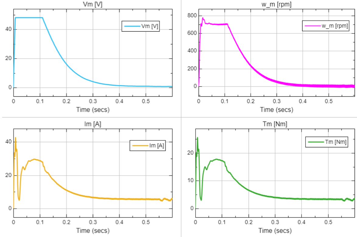
Figura 17: Variables eléctricas y mecánicas del motor ante referencia trapezoidal de 35^\circ
