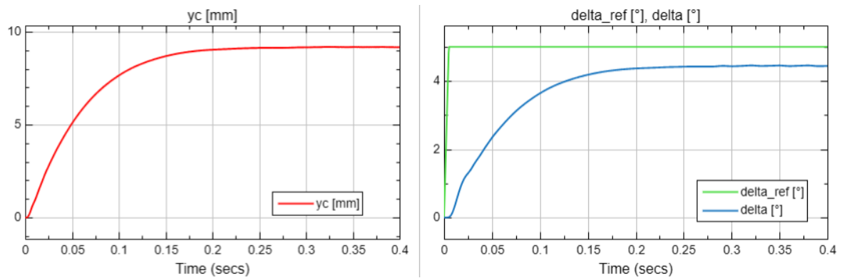
Figura 19: Respuesta \delta(t) y y_c(t) ante una referencia trapezoidal de 5^\circ
