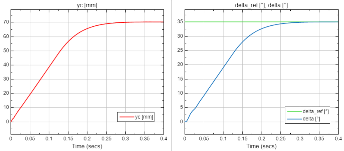
Figura 12: Respuesta \delta(t) y y_c(t) ante una referencia escalón de 35^\circ
