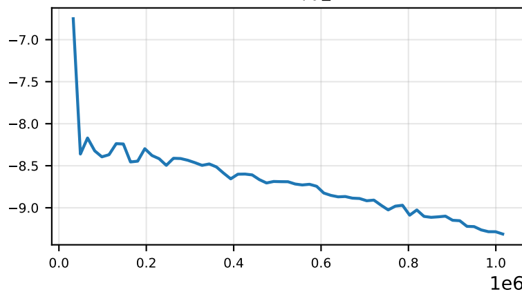
train/policy_gradient_loss
