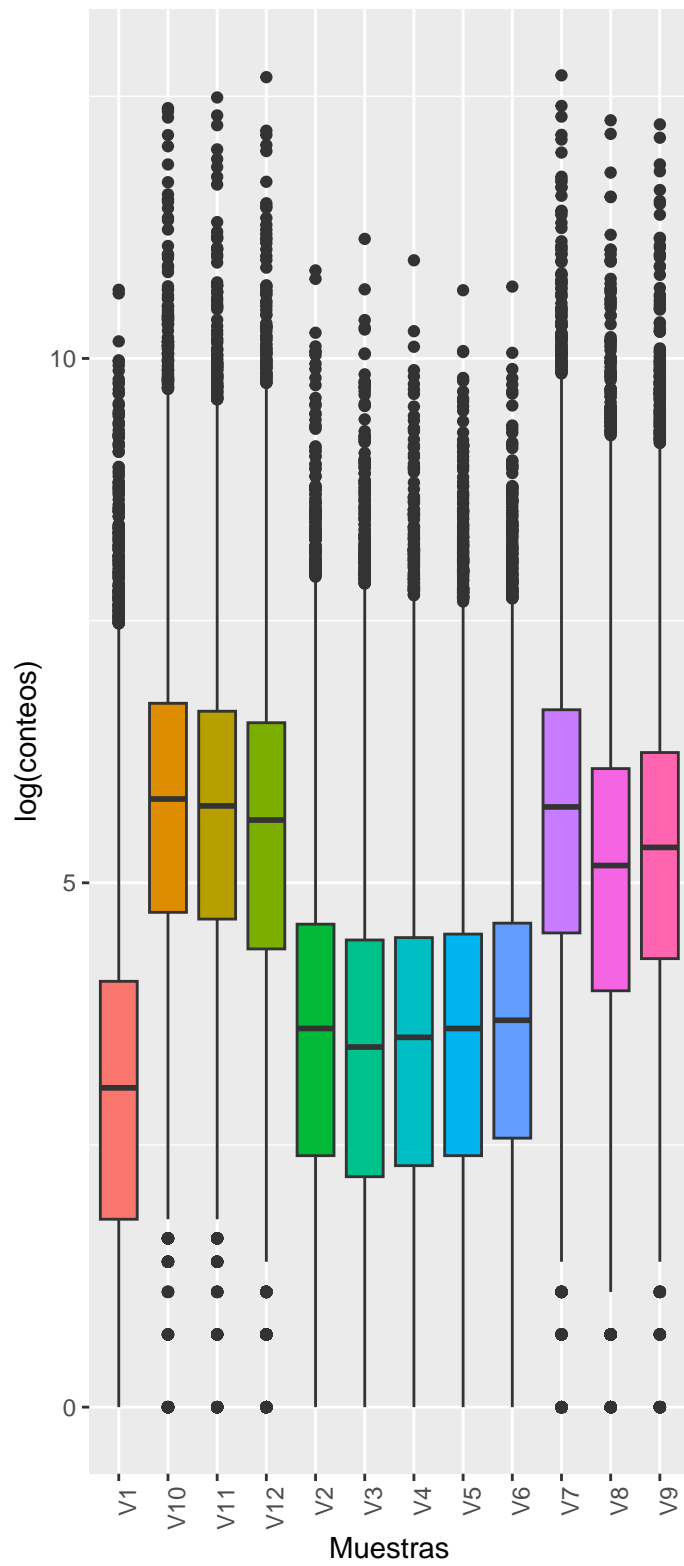
A Boxplot de conteos crudos
