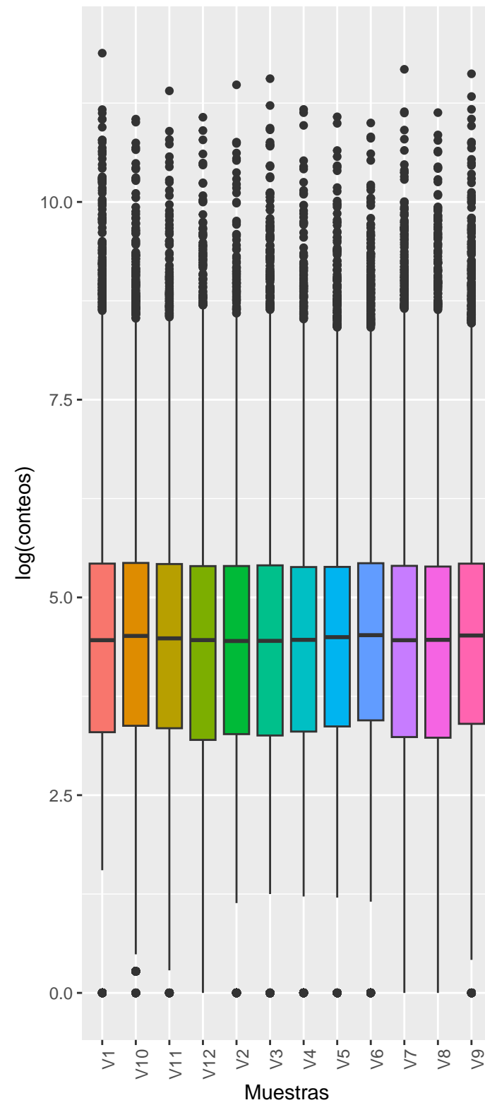
C Boxplot de conteos normalizados
