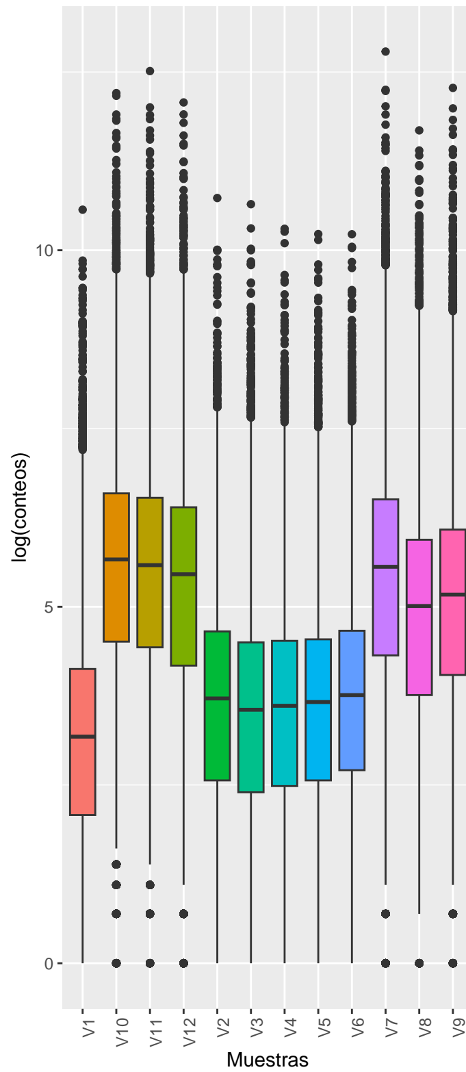
B Boxplot de conteos ajustados
