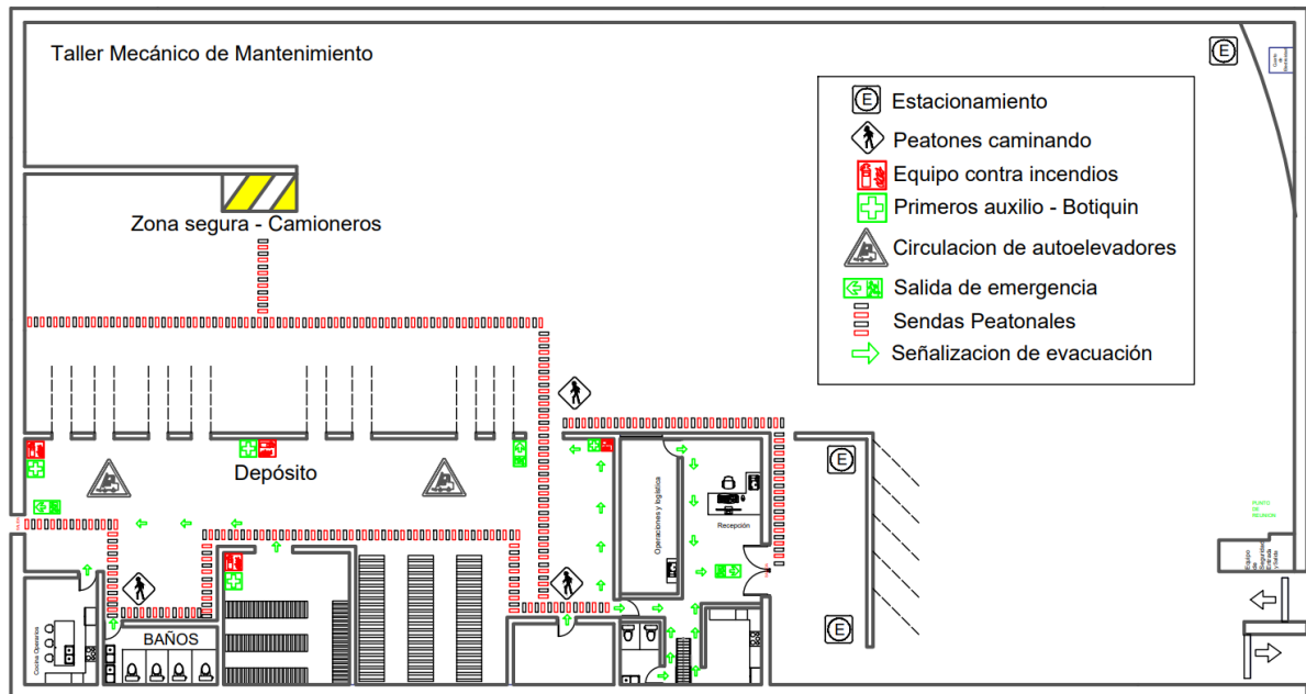
Ilustración 1: PlantaBaja
